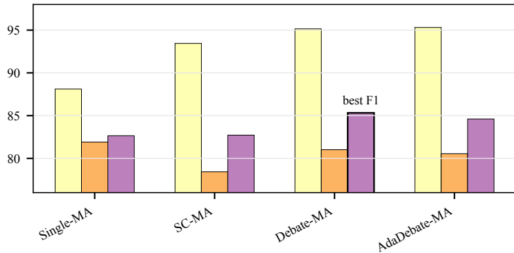
Answer-Set P/R/F1
