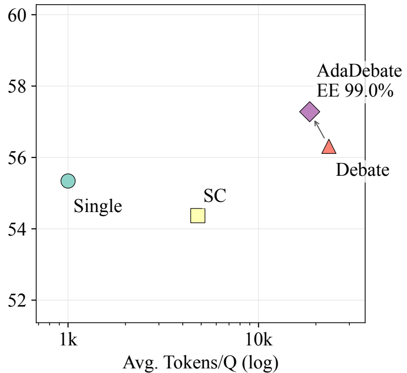
MultiRC (N=950)
