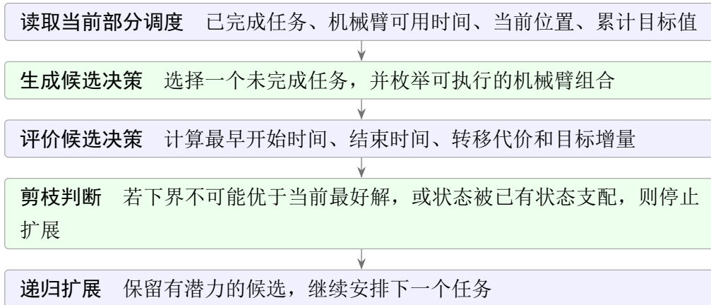
图 3: 自编隐枚举精确搜索的决策流程
