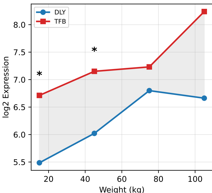
HGD
