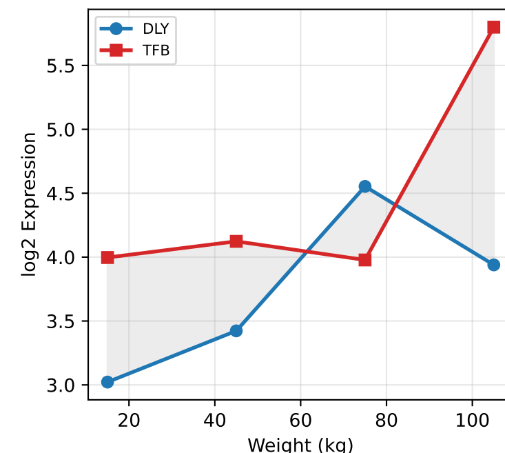
AASS
