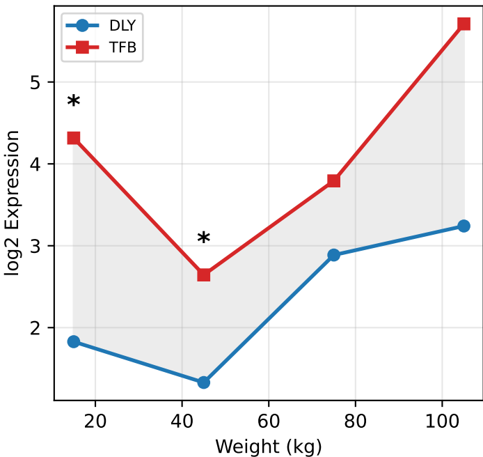
SDS
