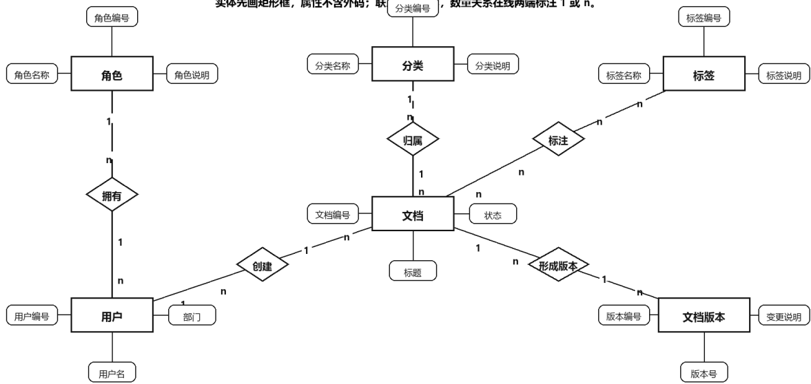
图 4-1：基础知识管理域 E-R 图
