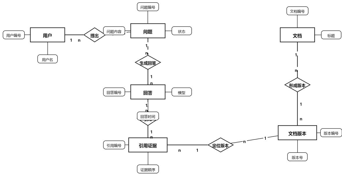
图 4-2：问答与版本追溯域 E-R 图
