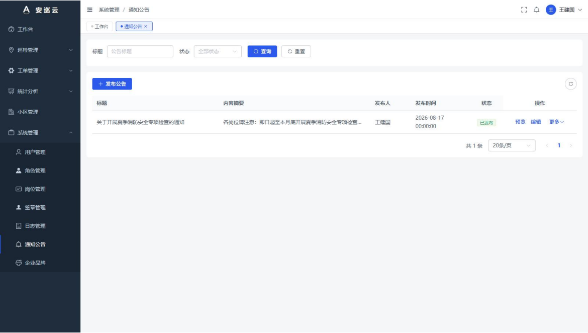
图 3-16 通知公告
