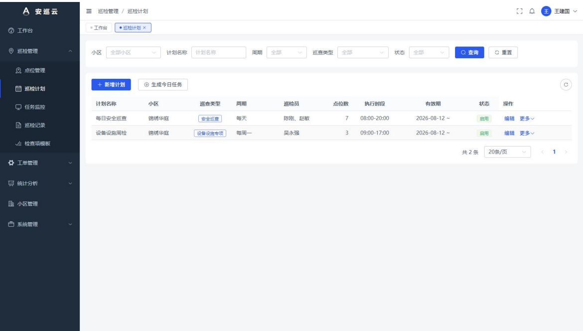
图 3-9 巡检计划
