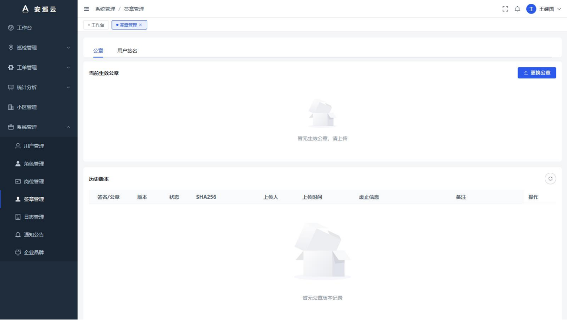
图 3-15 签章管理
