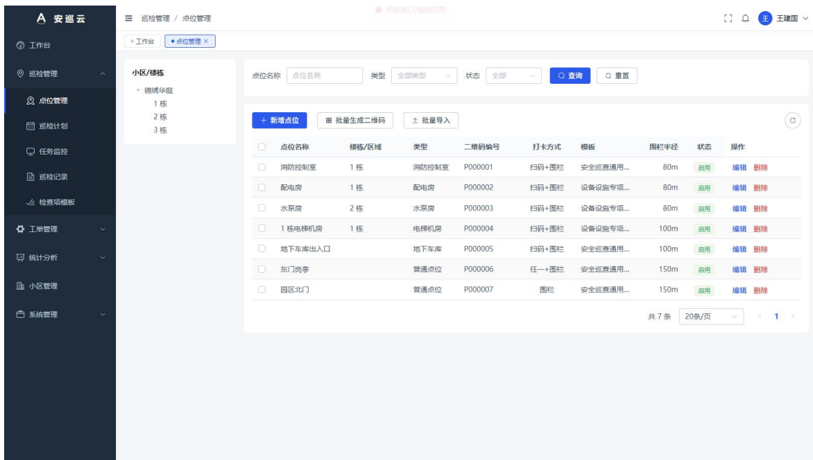
图 3-8 点位管理
