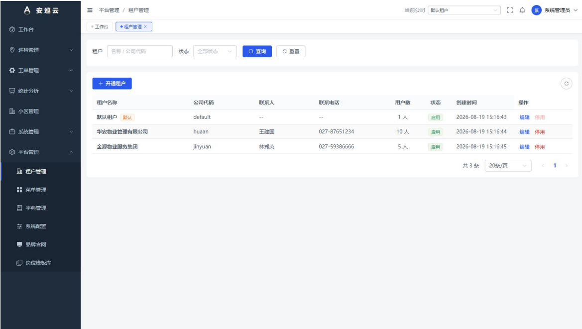
图 11-1 租户管理
