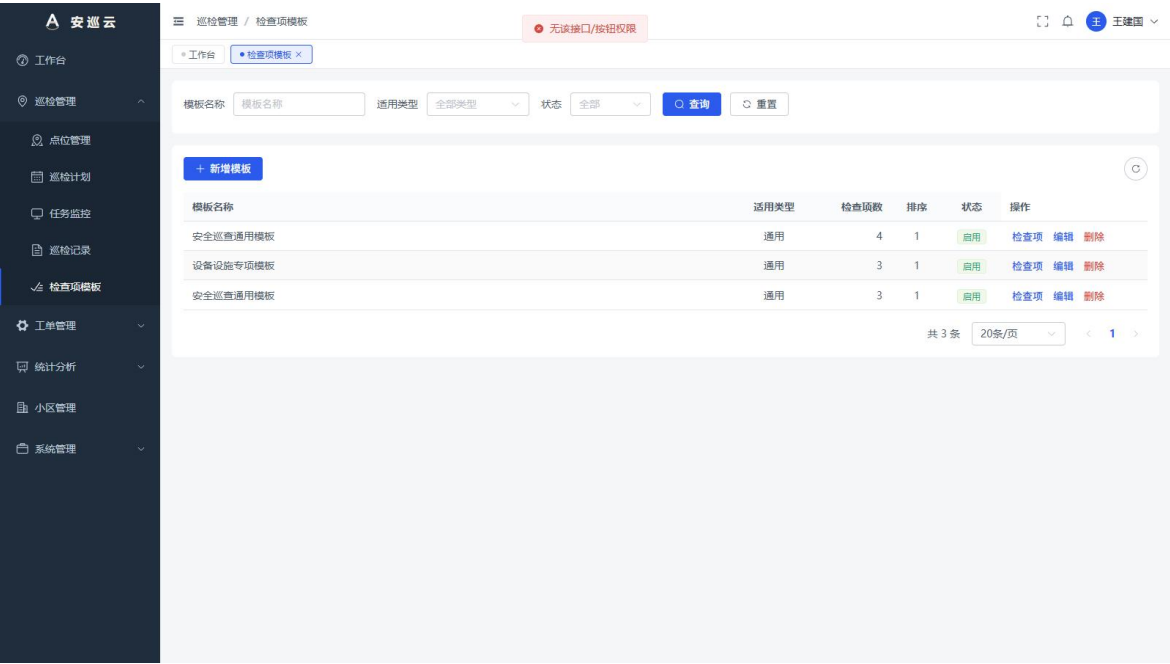
图 3-10 检查项模板
