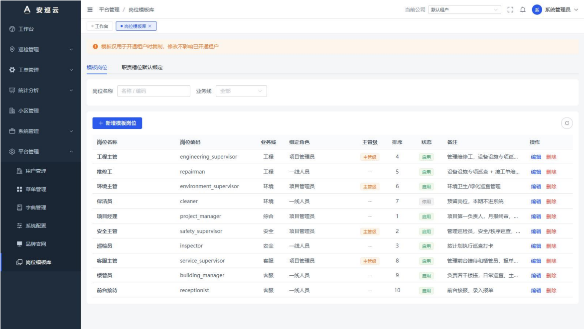
图 11-2 岗位模板库
