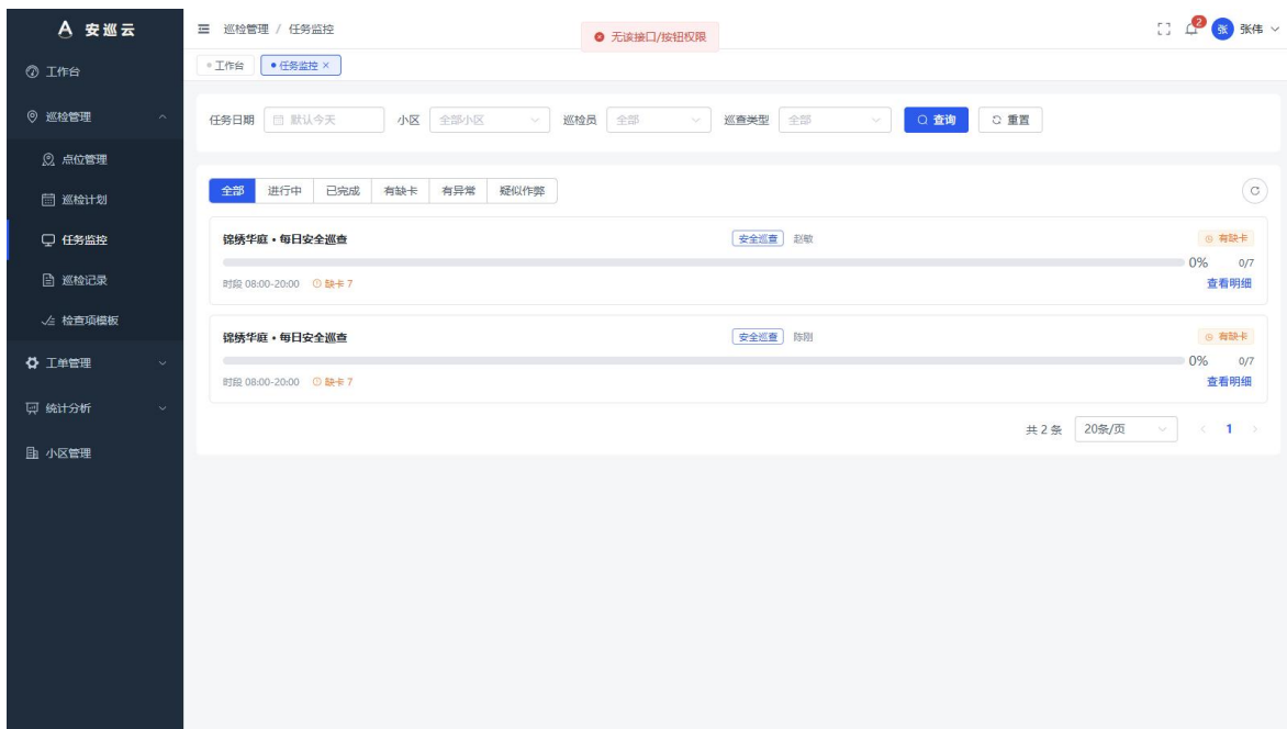
图 4-2 任务监控
