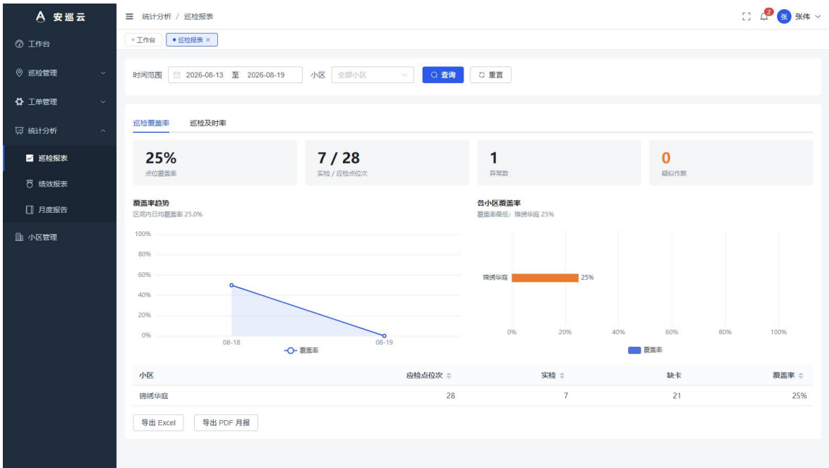
图 3-14 统计分析
