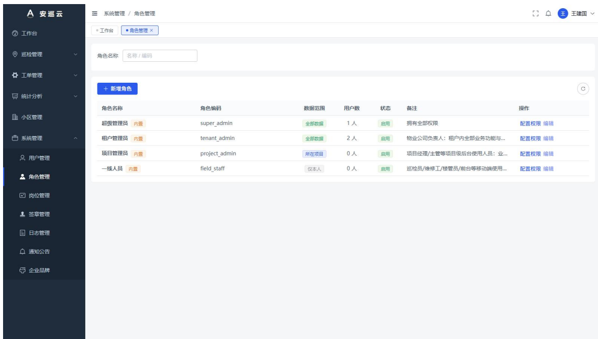
图 3-3 角色管理
