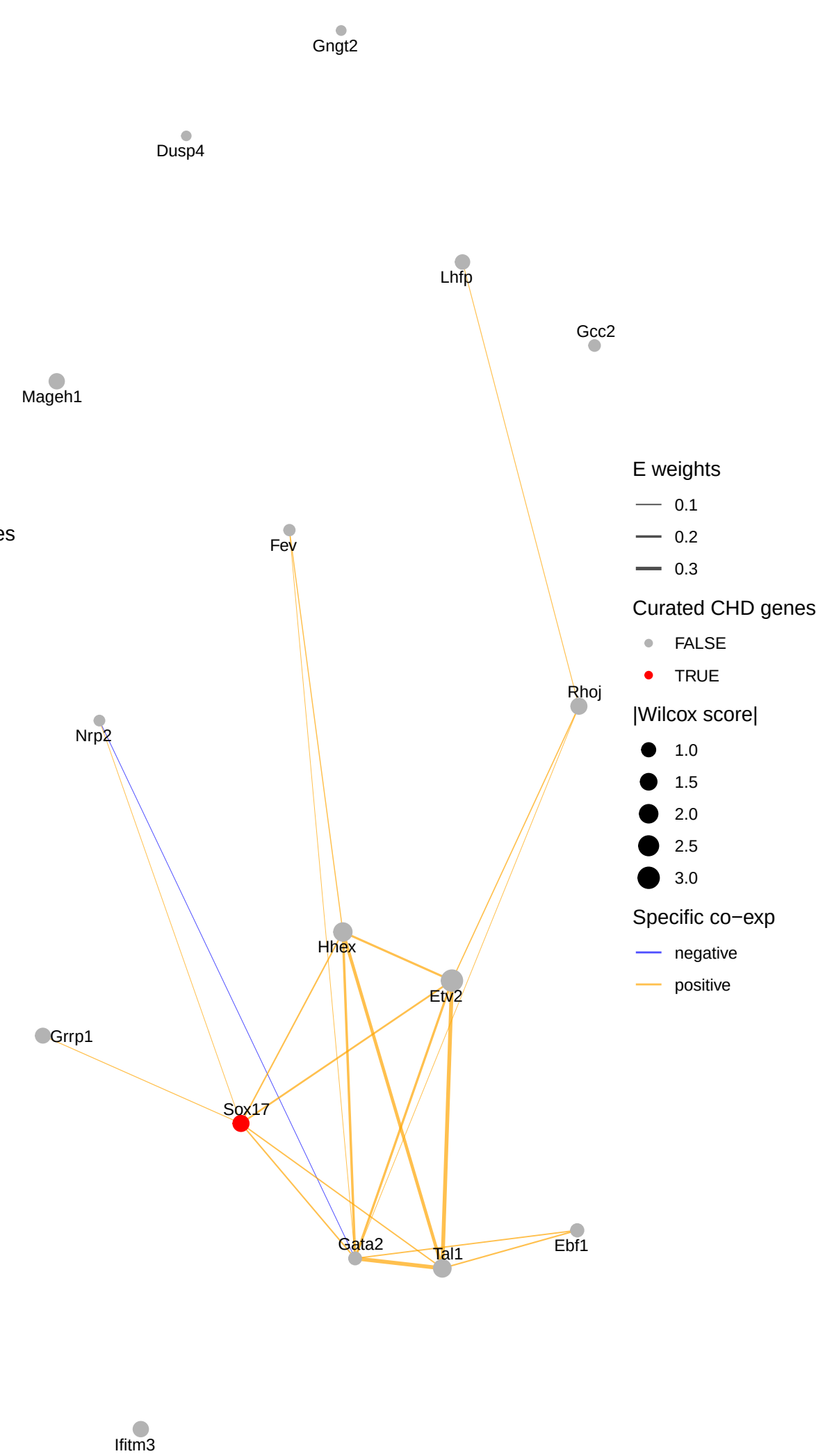
HiGCTS_endothelial.b 16 PPI genes
