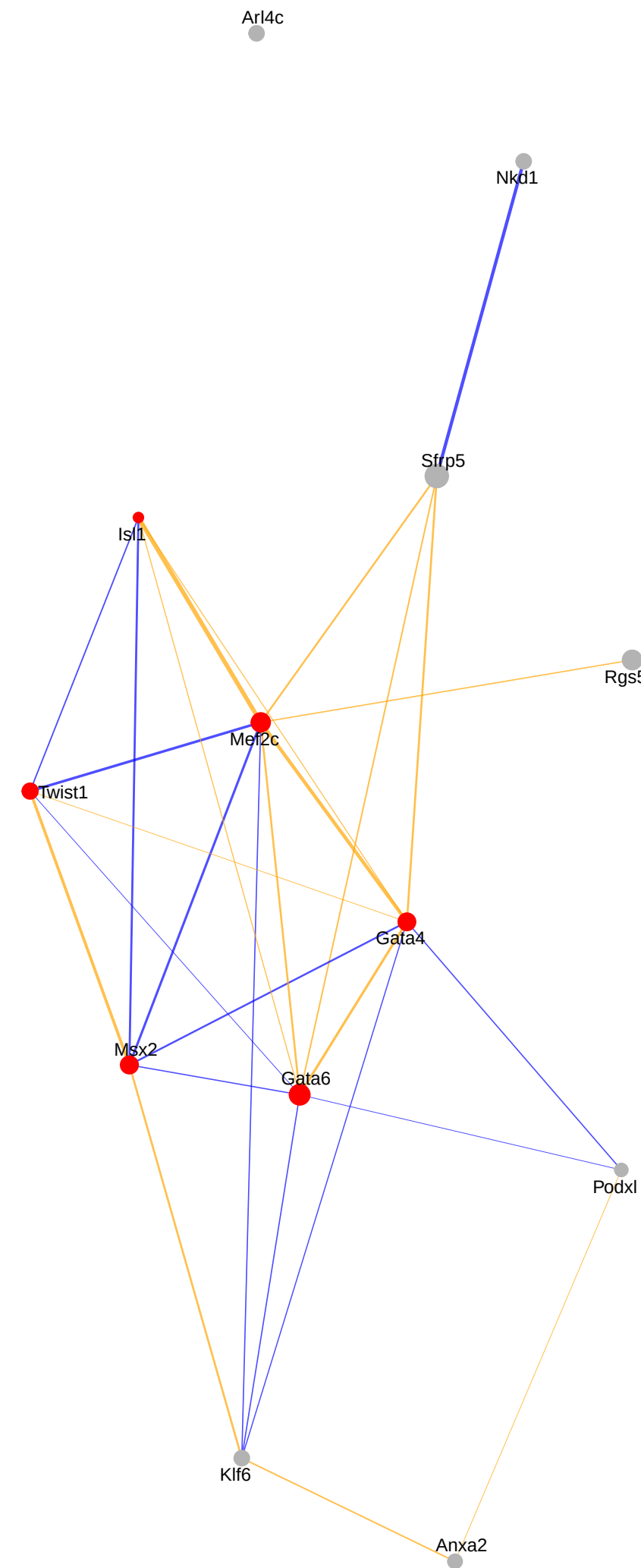
HiGCTS_cardiac.a 13 PPI genes
