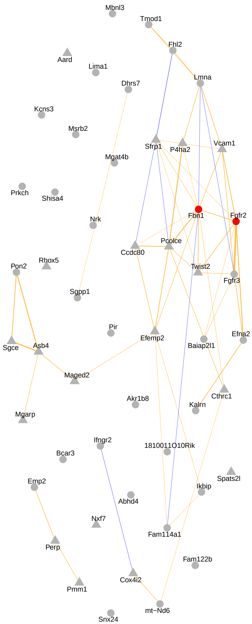
51 PPI genes
