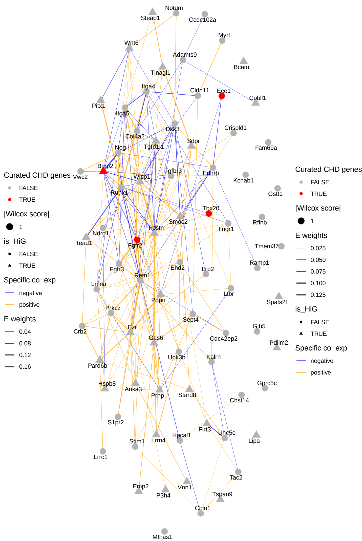
79 PPI genes
