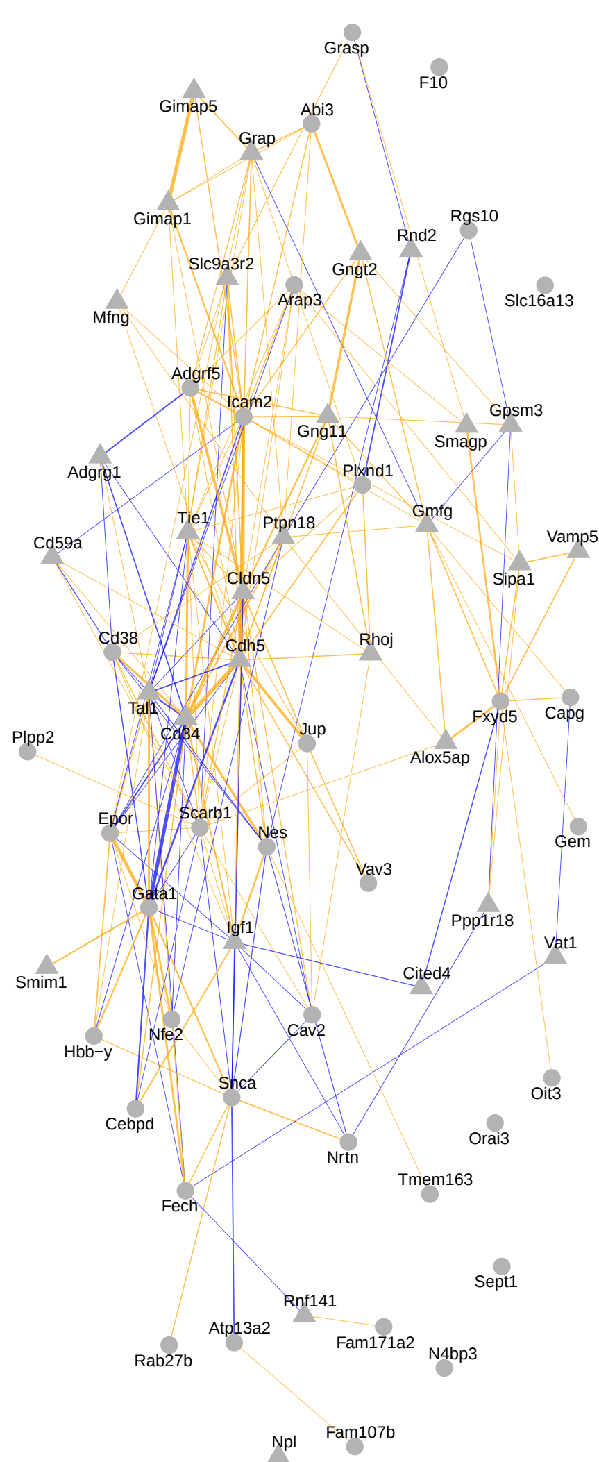
66 PPI genes
