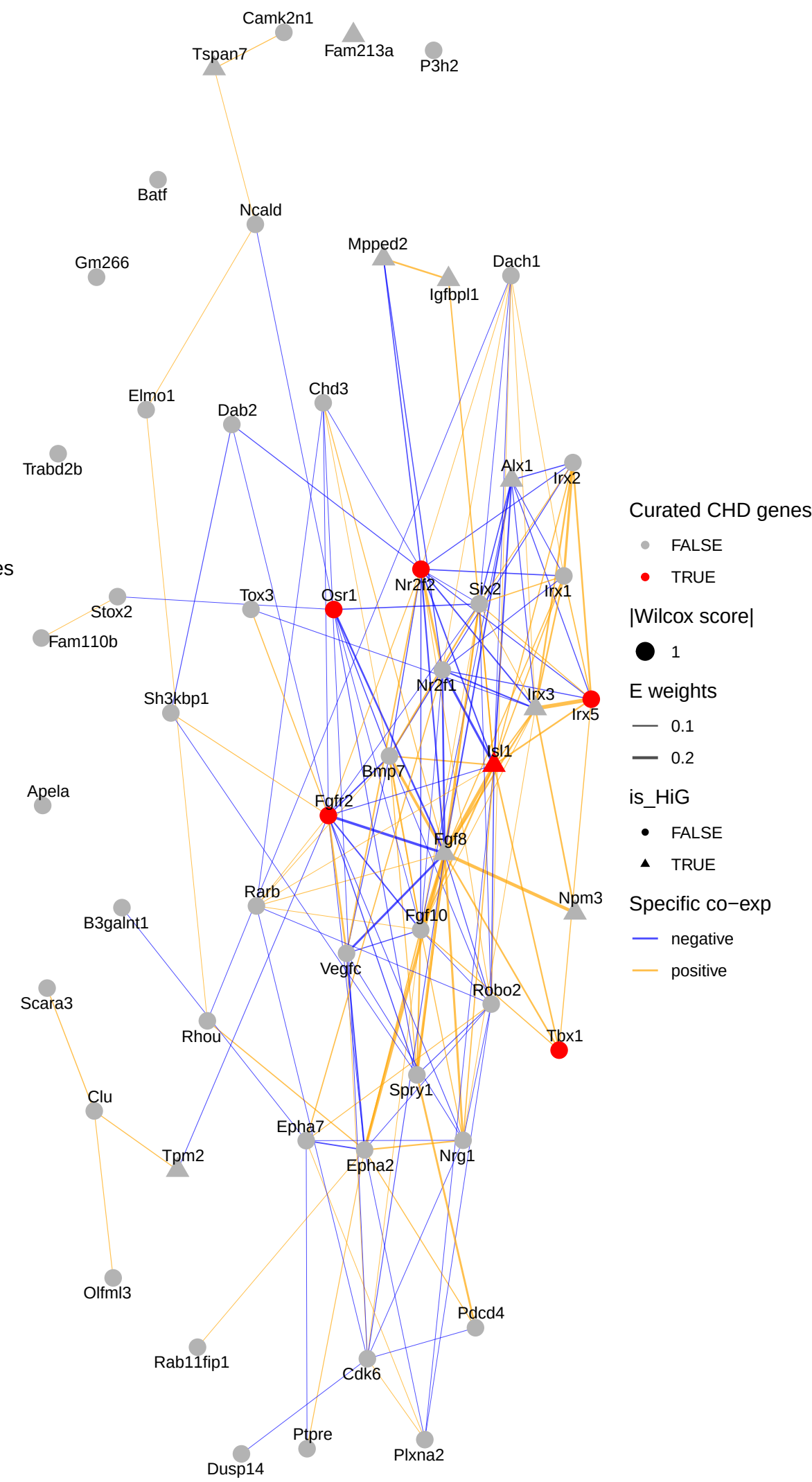
54 PPI genes
