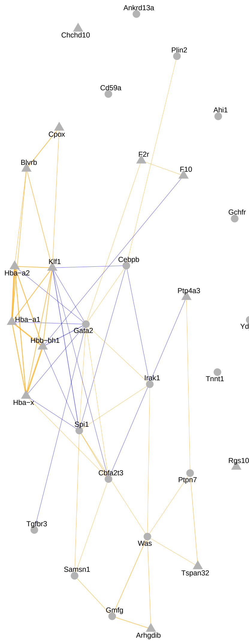
31 PPI genes
