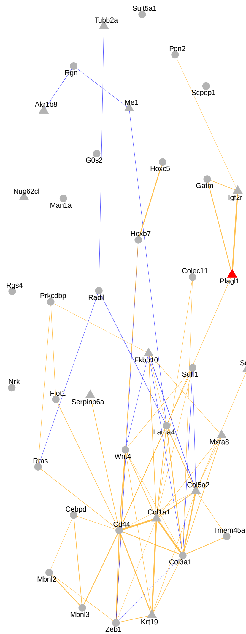
39 PPI genes
