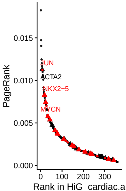
HiG_cardiac.a
