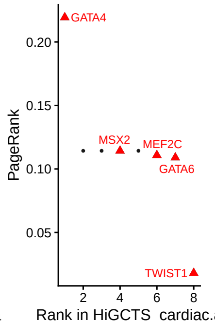
HiGCTS_cardiac.a
