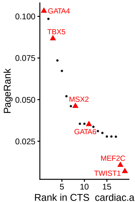
CTS_cardiac.a
