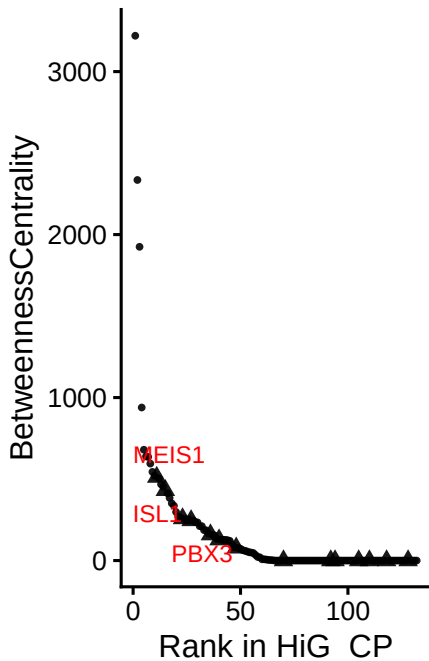
HiG_CP
