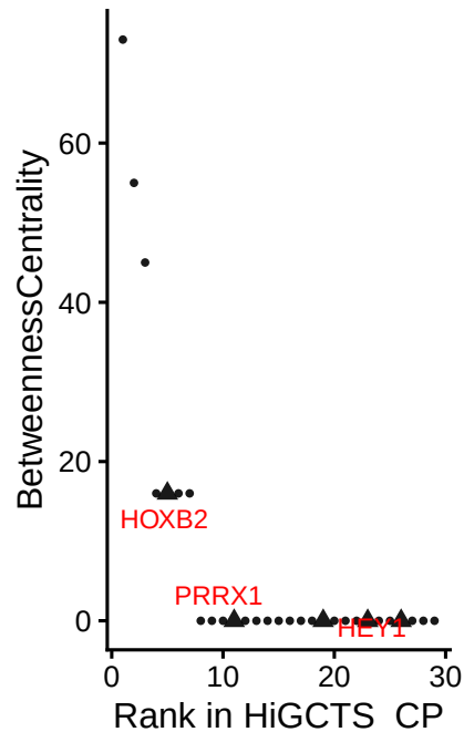
HiGCTS_CP
