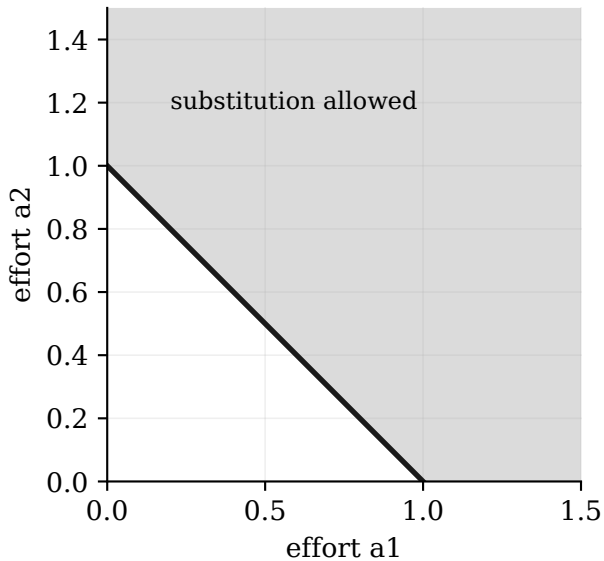
A. additive: a1 + a2 \geq t
