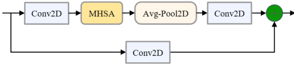
图 3.3 编码器结构
