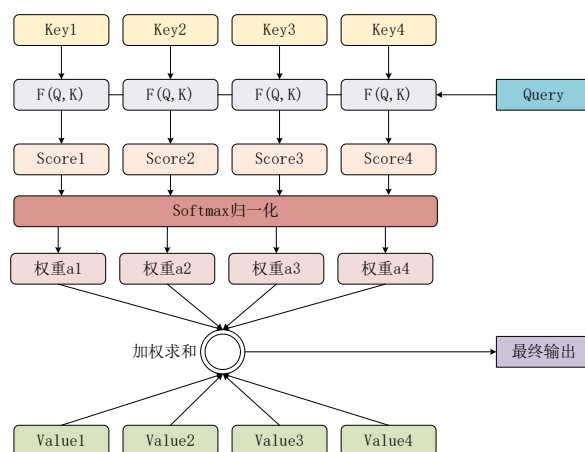
图 2.5 注意力机制处理过程
