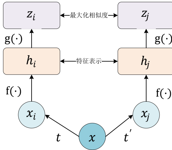
图 2.6 对比学习过程
