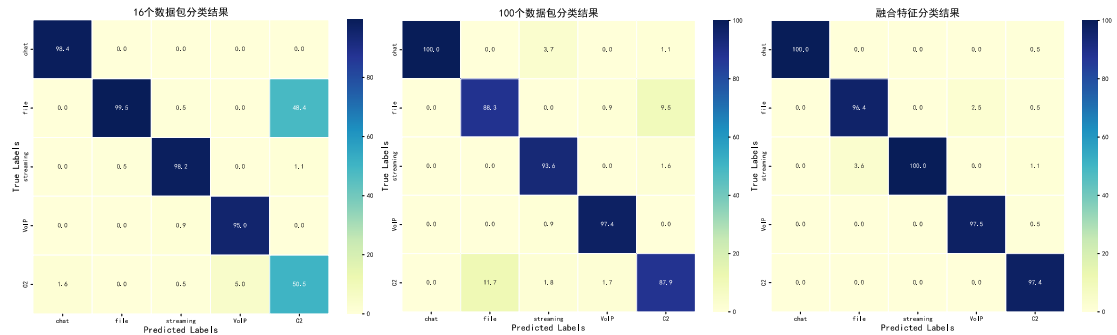
图 4.5 三种模型的混淆矩阵
