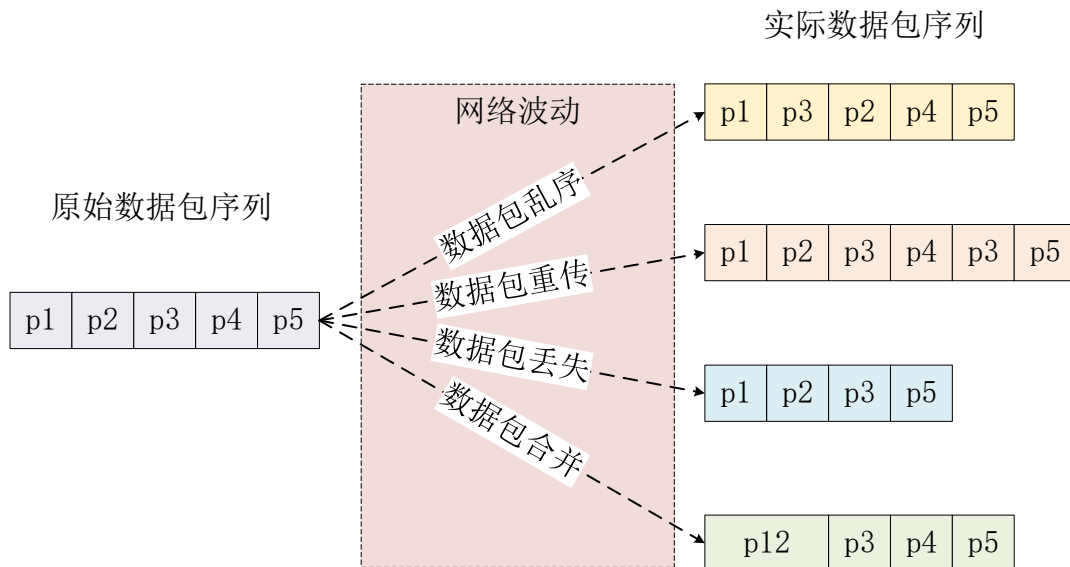
图 3.2 数据包序列变化
