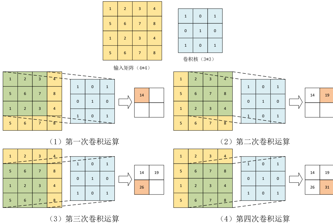
图 2.2 卷积运算过程
