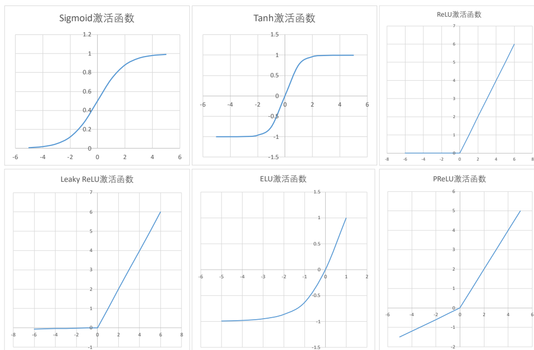
图 2.4 常见的激活函数图像
