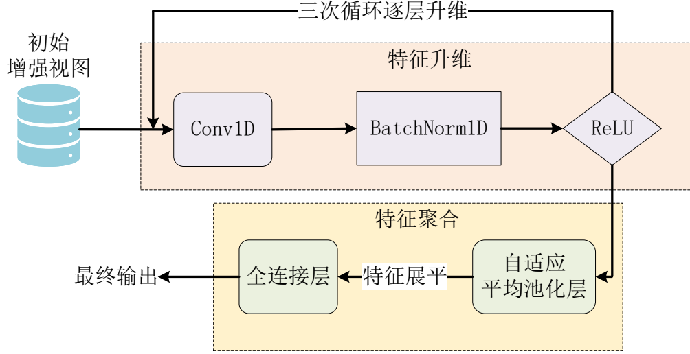
图 3.3 编码器结构
