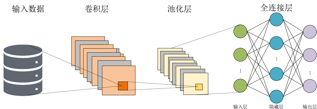
图 2.1 卷积神经网络结构
