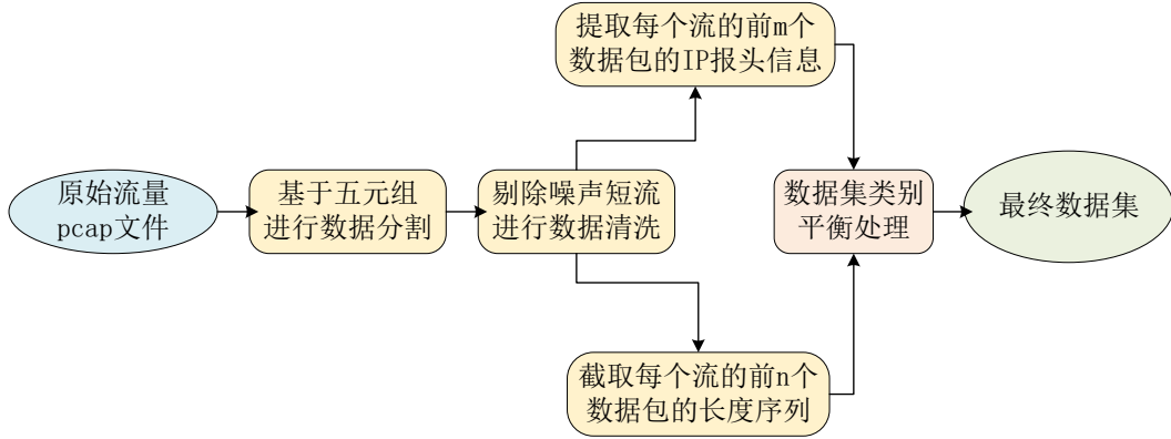
图 3.4 数据预处理流程
