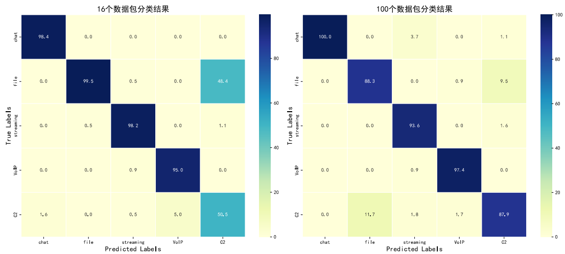
图 4.1 不同长度数据包序列分类结果混淆矩阵
