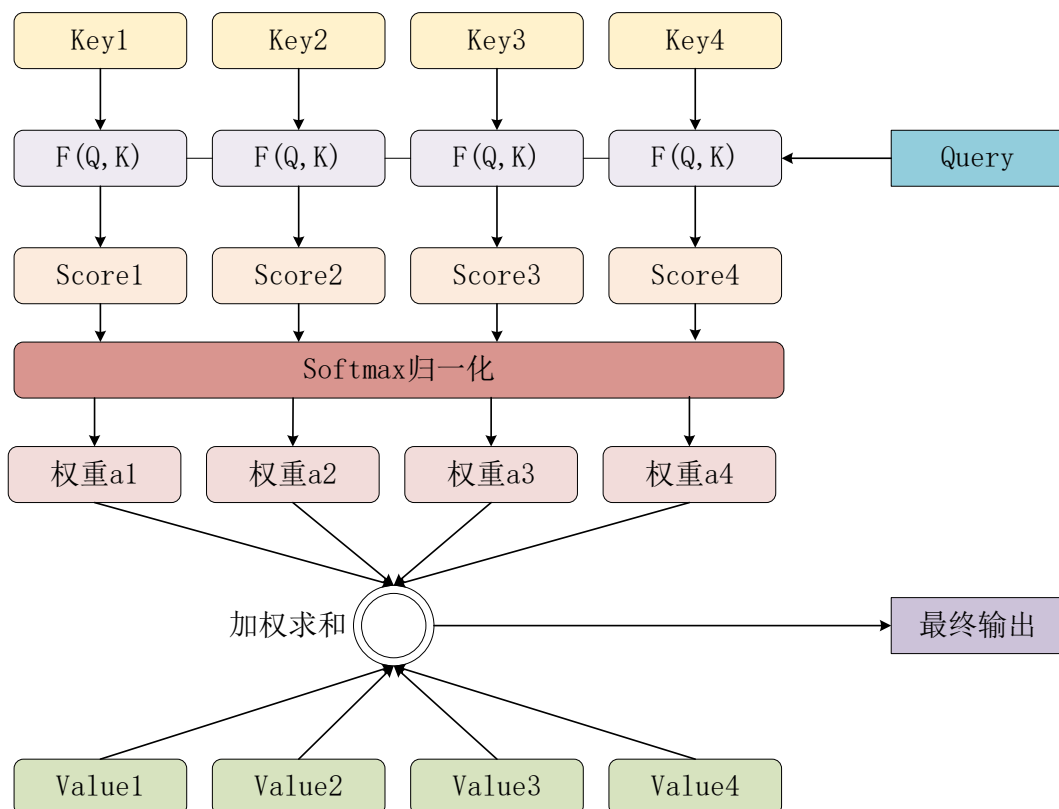
图 2.5 注意力机制处理过程
