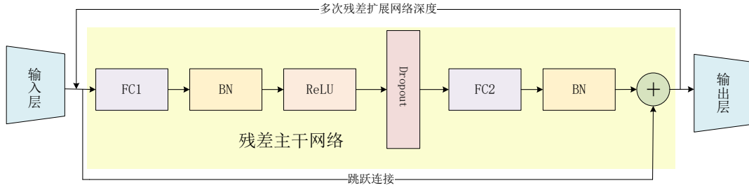
图 4.4 分类器结构
