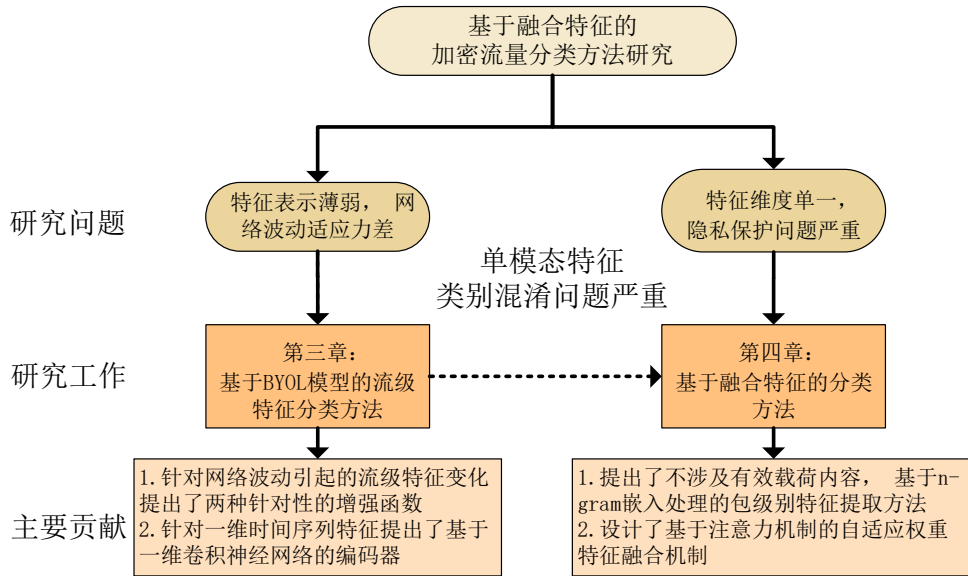
图 1.2 研究内容结构图
