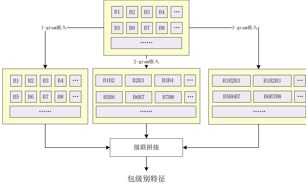
图 4.3 n-gram 嵌入处理
