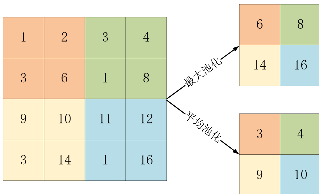
图 2.3 两种池化方式
