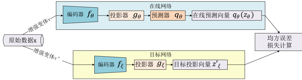
图 3.1 BYOL 模型框架
