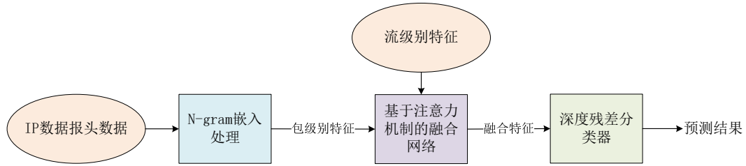
图 4.2 融合特征分类模型架构
