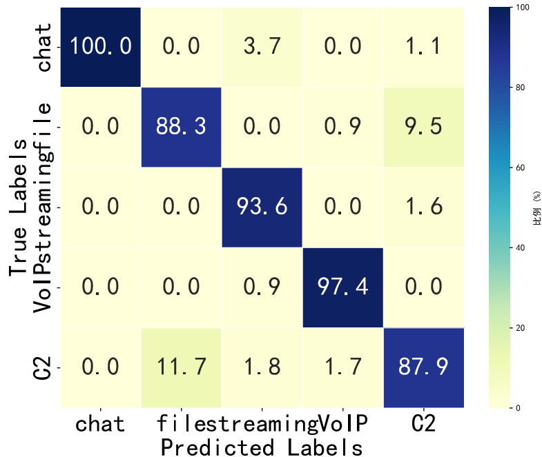
100个数据包分类结果
