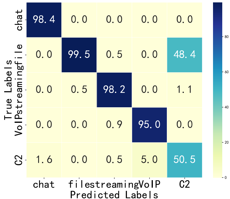
16个数据包分类结果
