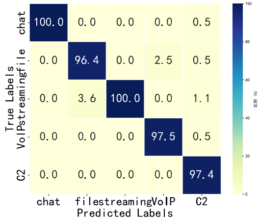
融合特征分类结果
