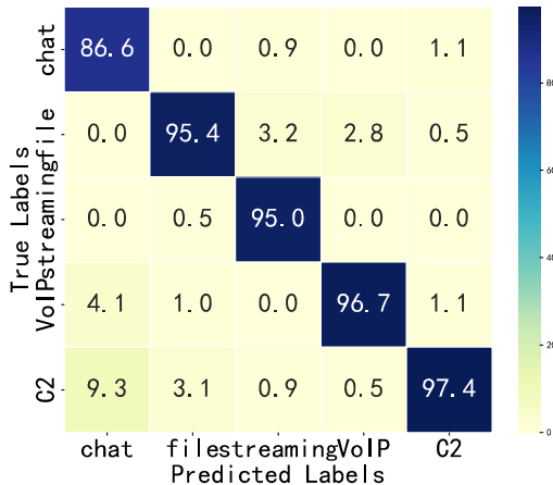
包级别特征分类结果
