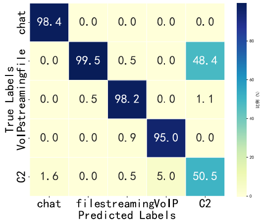
16个数据包分类结果
