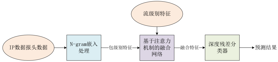
图 4.2 融合特征分类模型架构
