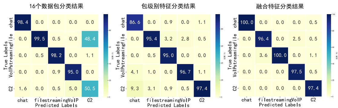
图 4.5 三种模型的混淆矩阵
