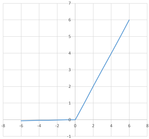
Leaky ReLU激活函数
