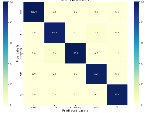
融合特征分类结果
