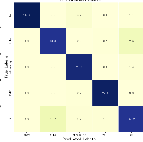
100个数据包分类结果
