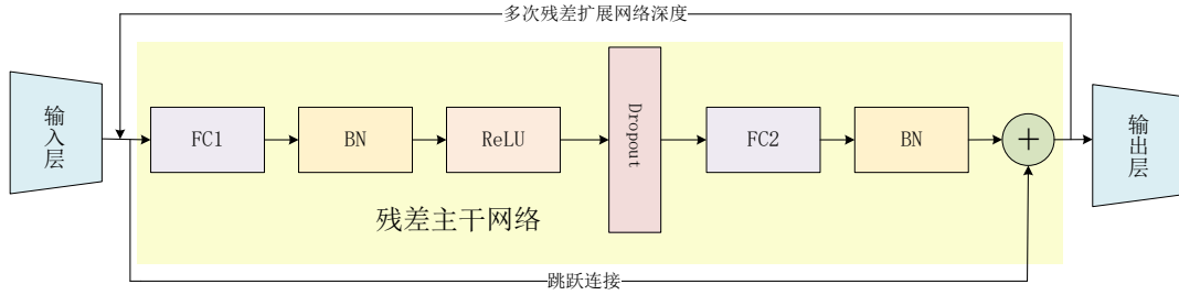
图 4.4 分类器结构
