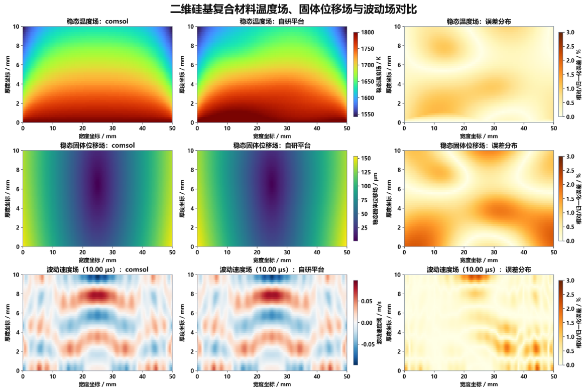
图 3.21 二维硅基复合材料温度场、固体场与波动场
