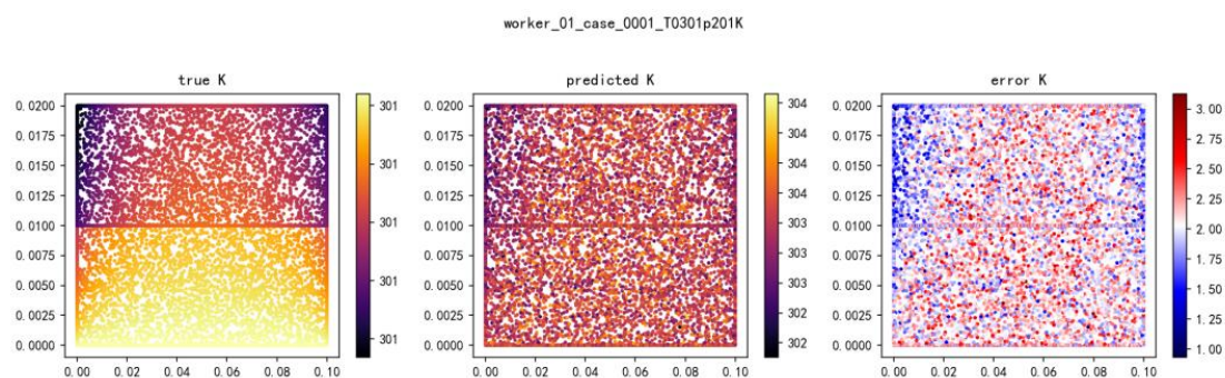
图 3.53 二维稳态实验测温验证结果
