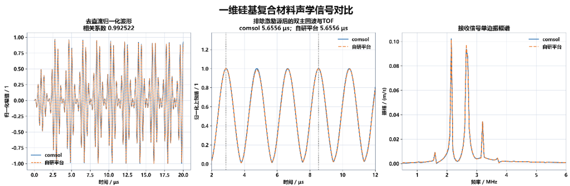
图 3.22 一维硅基复合材料声学波形及主回波
