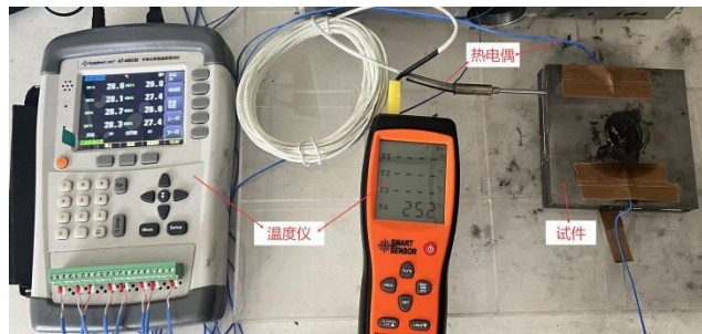
图 3.38 温度仪与试件连接实物图
