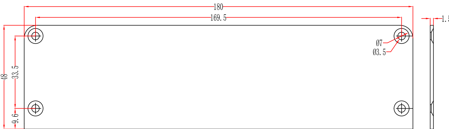
挡板
