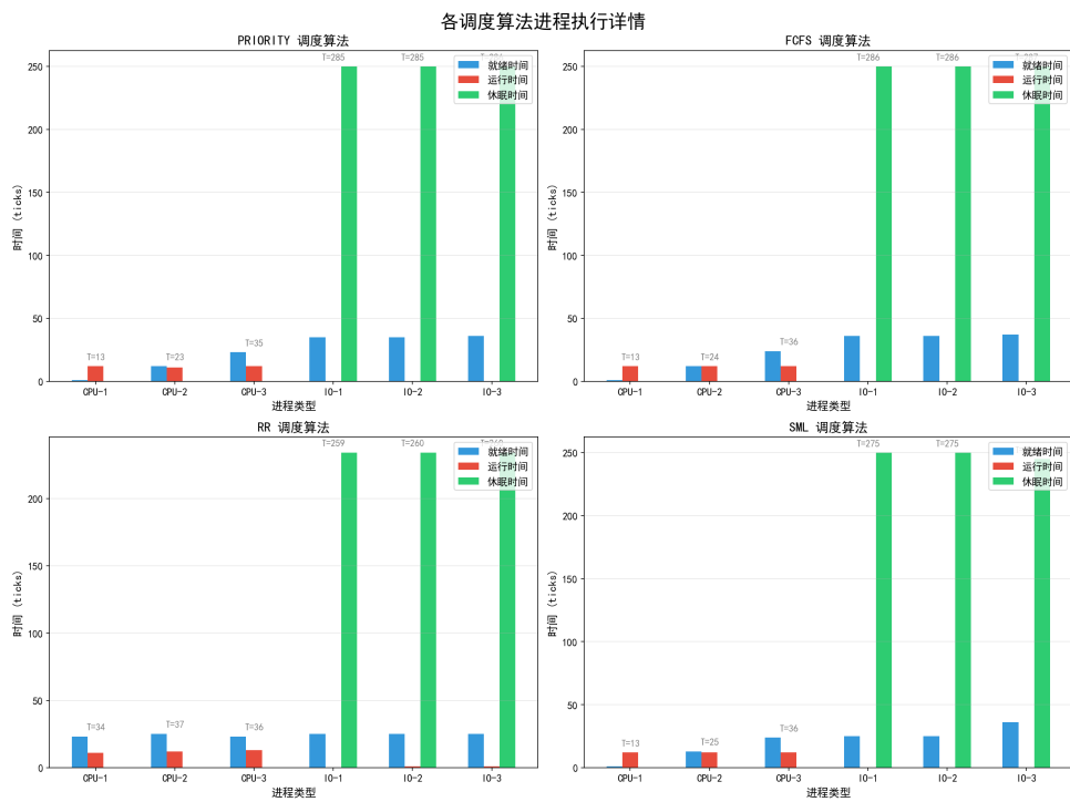
图 25 各进程执行详情
