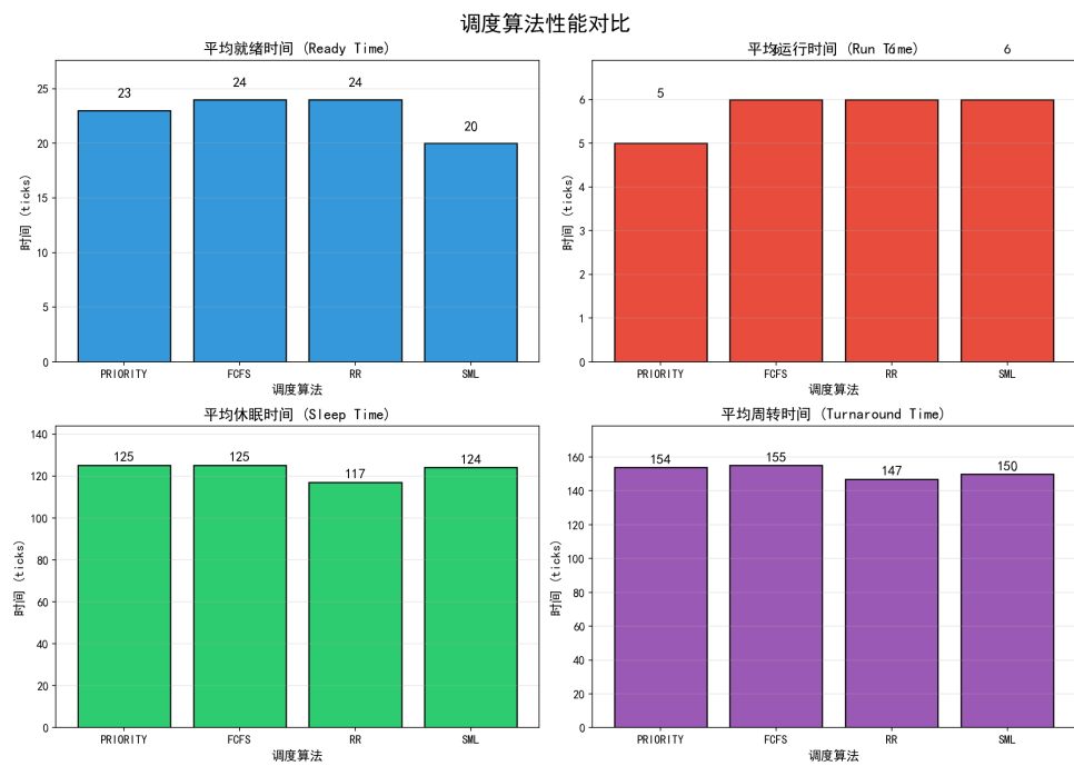
图 24 平均性能指标对比
