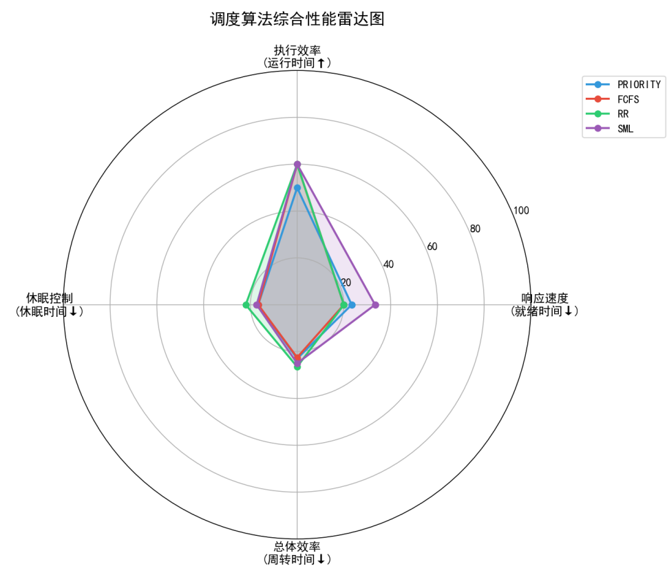
图 27 综合性能雷达图
