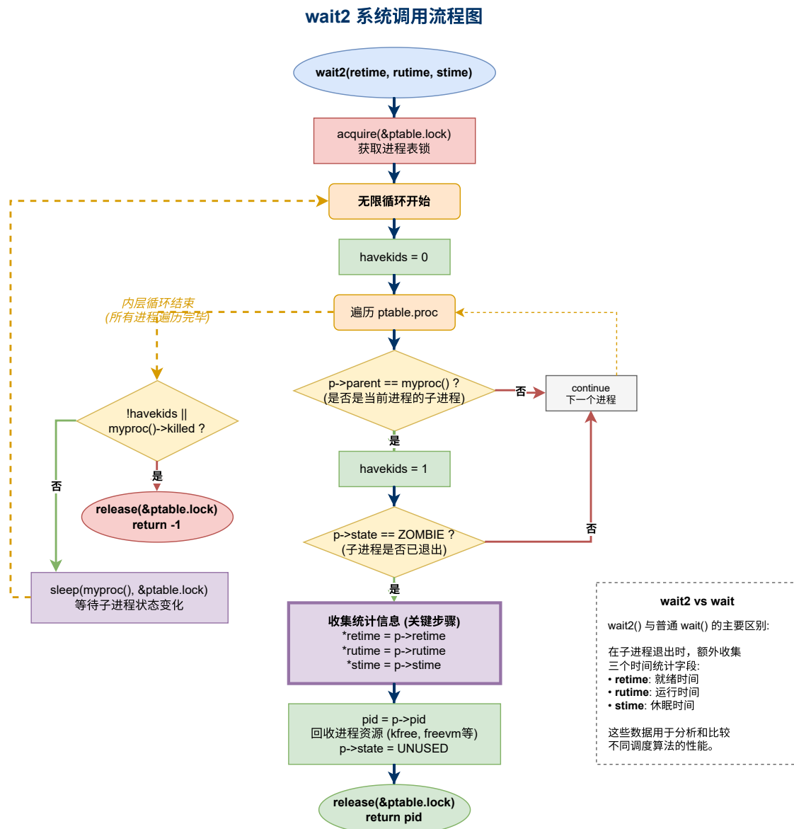
图 18 wait2 系统调用实现流程
