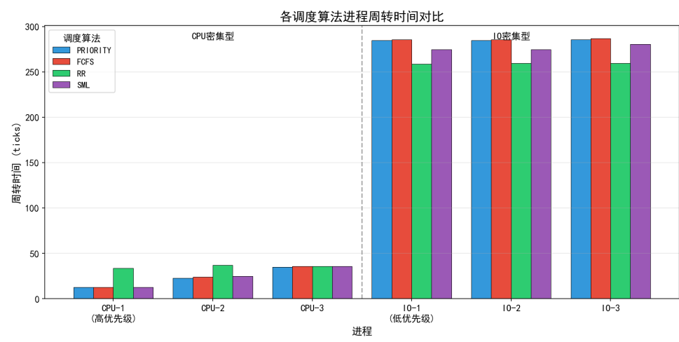
图 26 周转时间对比
