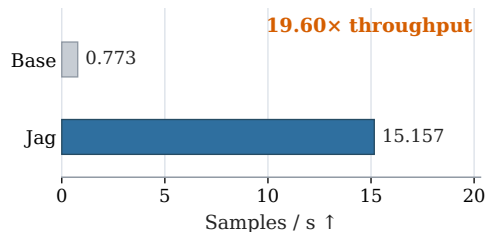
(d) Prediction throughput
