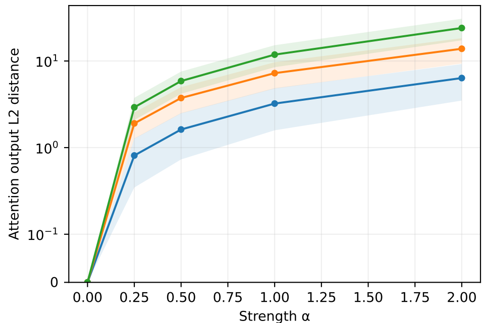
Lemma 8 · Layer 17 (zero-based) · prediction step 128
