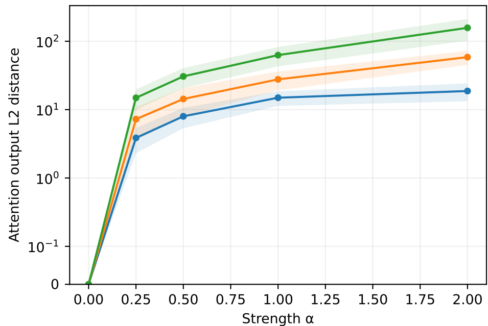
Lemma 8 · Layer 26 (zero-based) · prediction step 128
