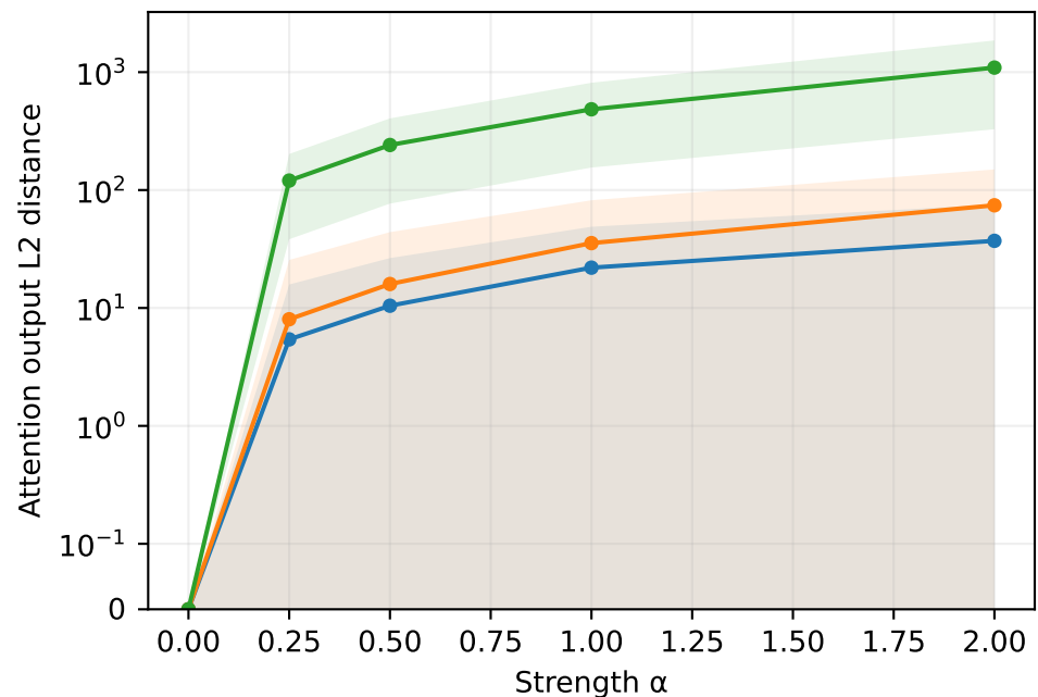
Lemma 8 · Layer 33 (zero-based) · prediction step 128
