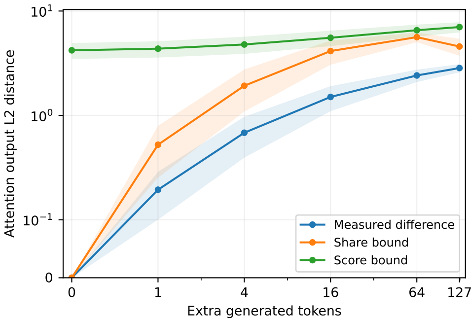
Lemma 8 · Layer 8 (zero-based) · prediction step 128
