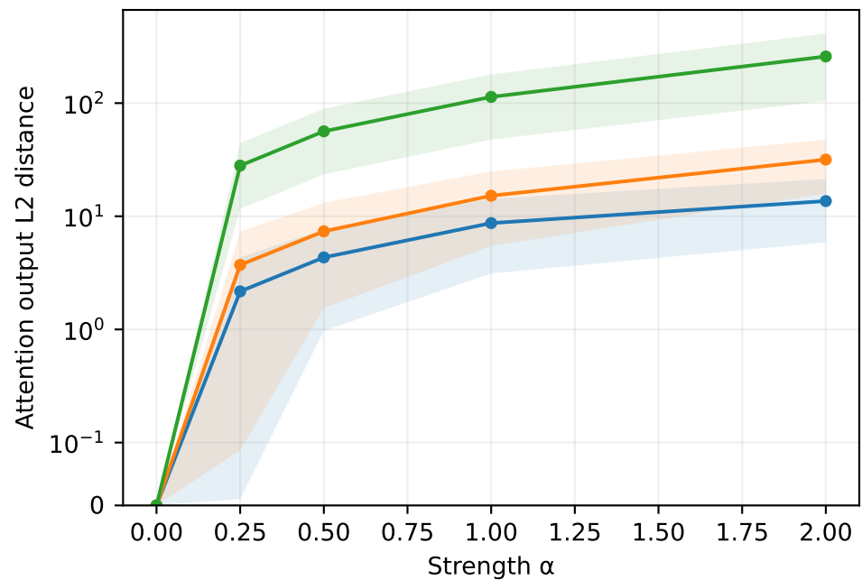
Lemma 8 · All layers · prediction step 128
