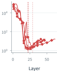
(b) Gemma
