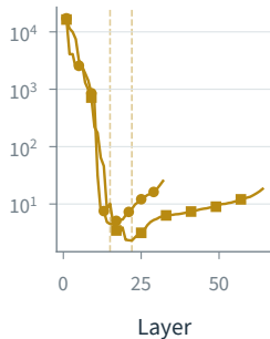
(c) OLMo-3
