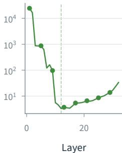
(d) Llama-3
