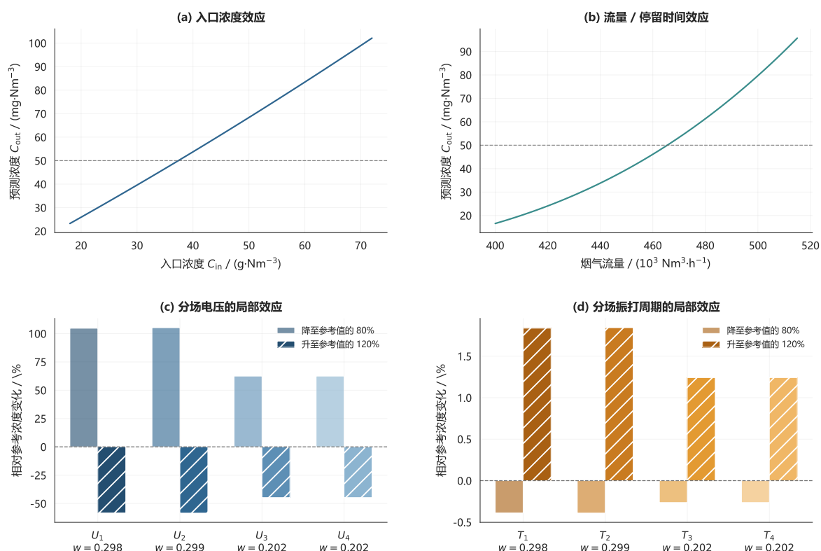
图 4 入口条件响应曲线及电压、振打周期的分场局部效应
