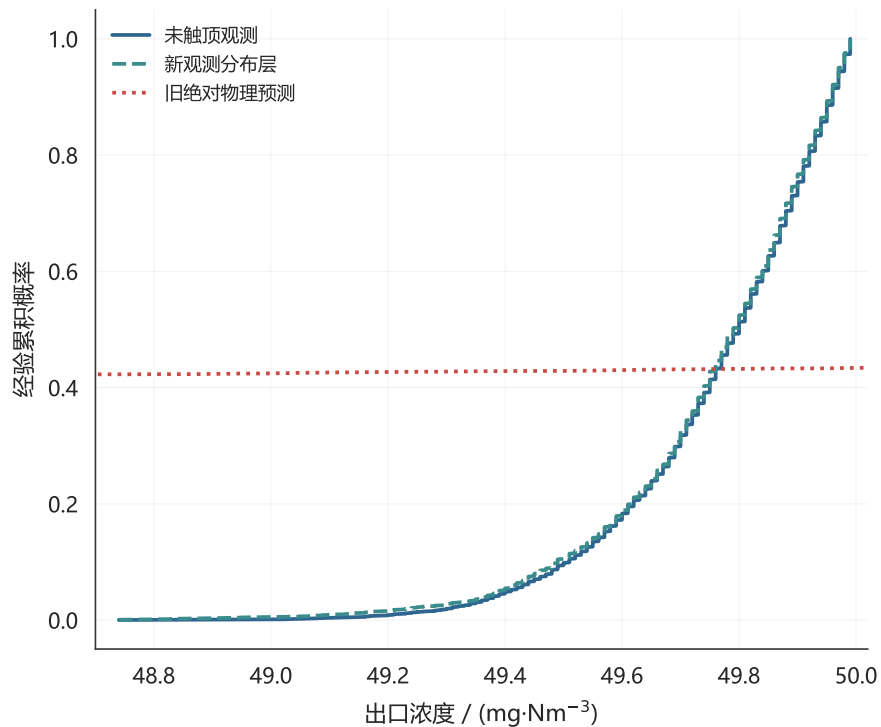
(b) 量程以下分布的局部比较
