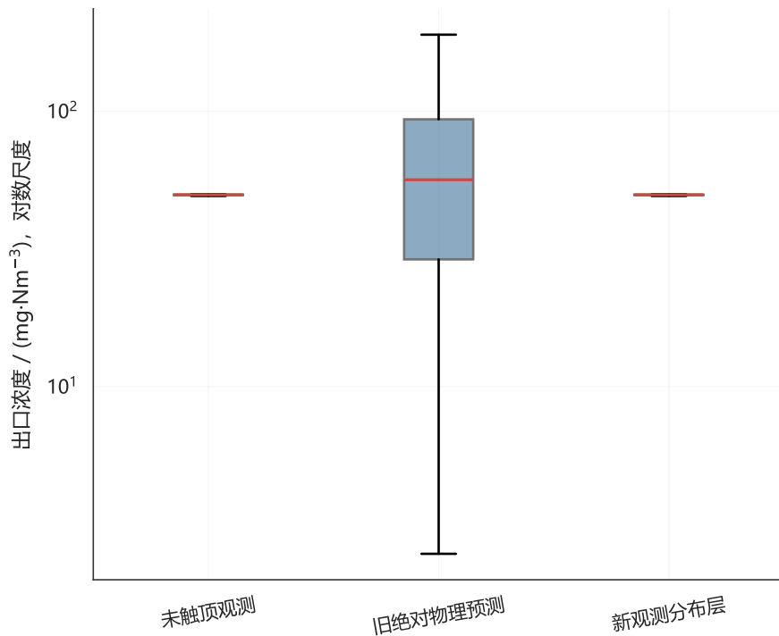
(a) 预测分布尺度比较
