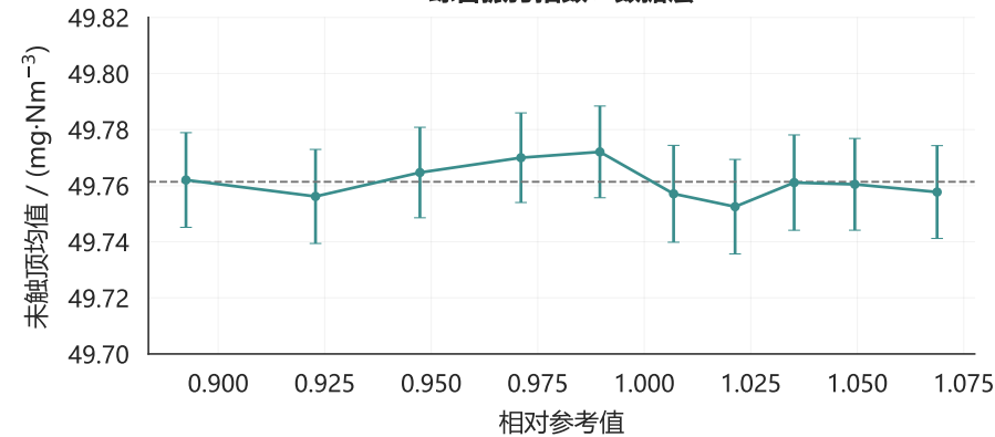
综合振打指数：数据层
