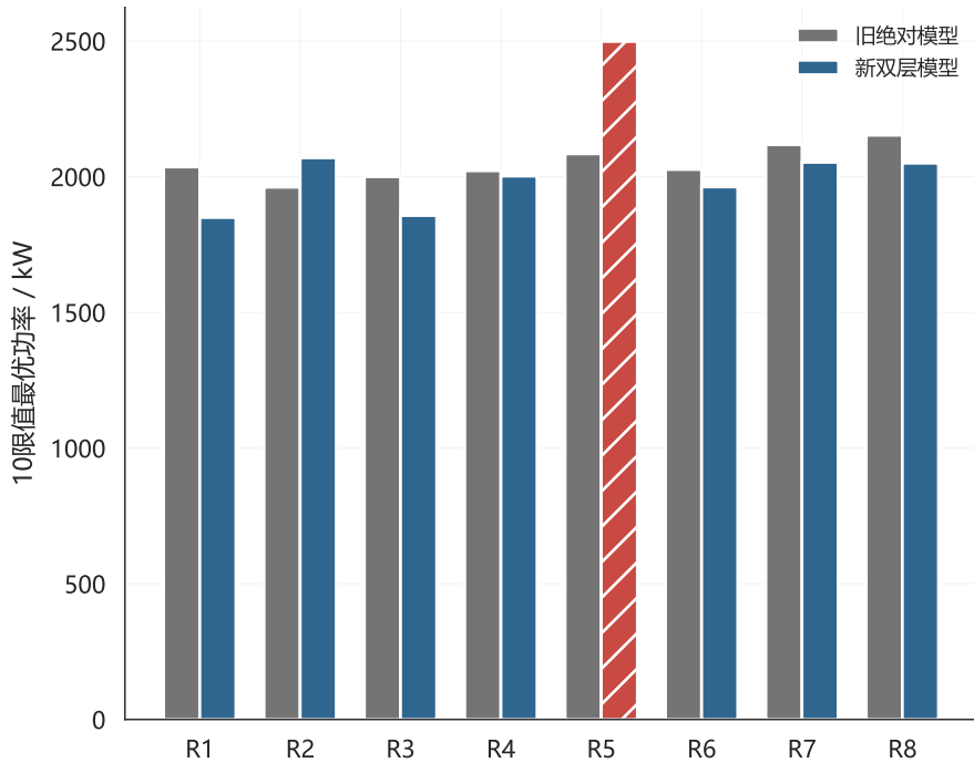
(a) 各工况10限值功率
