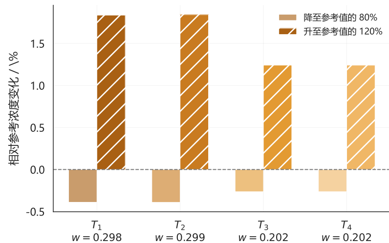
(d) 分场振打周期的局部效应
