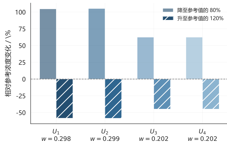
(c) 分场电压的局部效应
