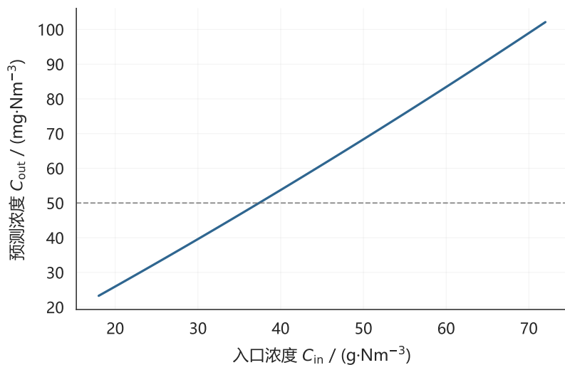
(a) 入口浓度效应
