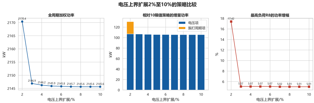
图 13 电压上界由历史上界的 102% 放宽至 110% 时的策略变化
