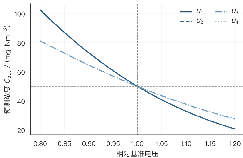
(c) 分场电压单调效应
