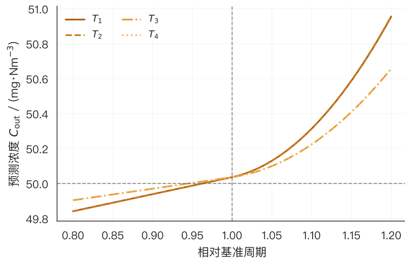
(d) 振打周期的积灰-再飞扬折中
