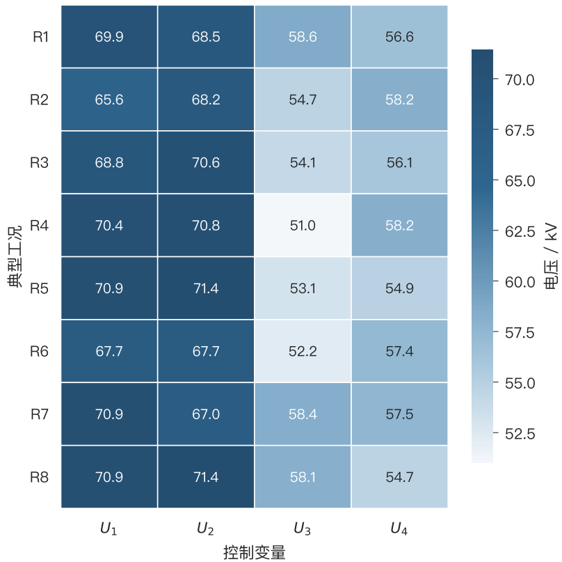
(a) 四电场电压
