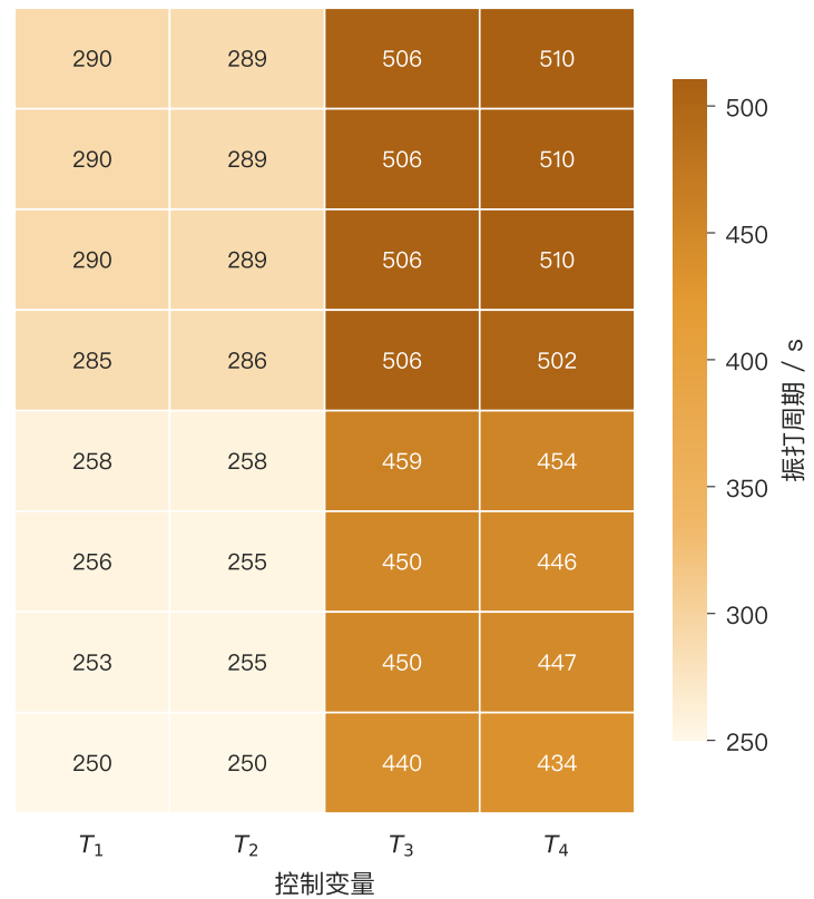
(b) 四电场振打周期
