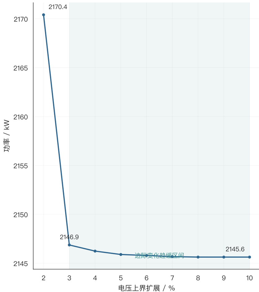
(a) 全周期加权功率
