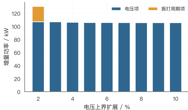
(b) 相对 10 \text{ mg} \cdot \text{Nm}^{-3} 策略的增量功率
