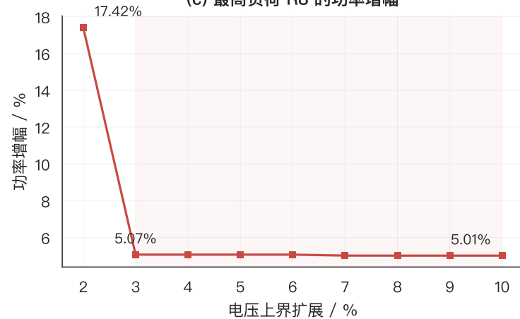
(c) 最高负荷 R8 的功率增幅
