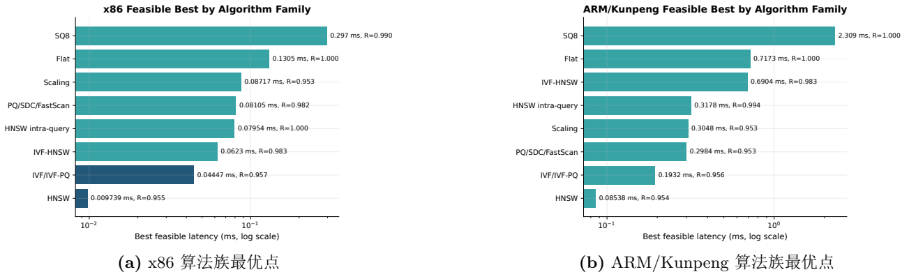
图 3: x86 与 ARM/Kunpeng 平台各算法族在 recall@100 \geq 0.95 下的最优可行点。两张图使用同一评价口径，便于观察算法结构是否跨平台保持一致。
