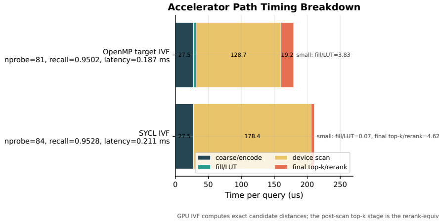
图 8: OpenMP target 与 oneAPI/SYCL 的阶段耗时分解。GPU IVF 已在设备端计算候选精确距离, 因此图中 final top-k/rerank 表示扫描后的最终重排阶段。
