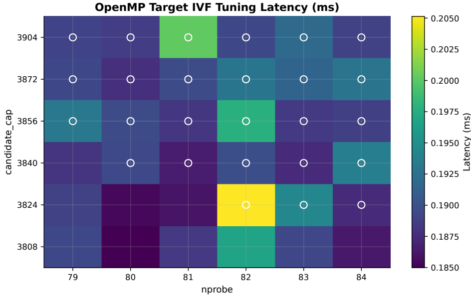
图 7: OpenMP target IVF 的 nprobe 与 candidate cap 调参热力图。白色圆圈为跨过目标 recall 线的可行点。
