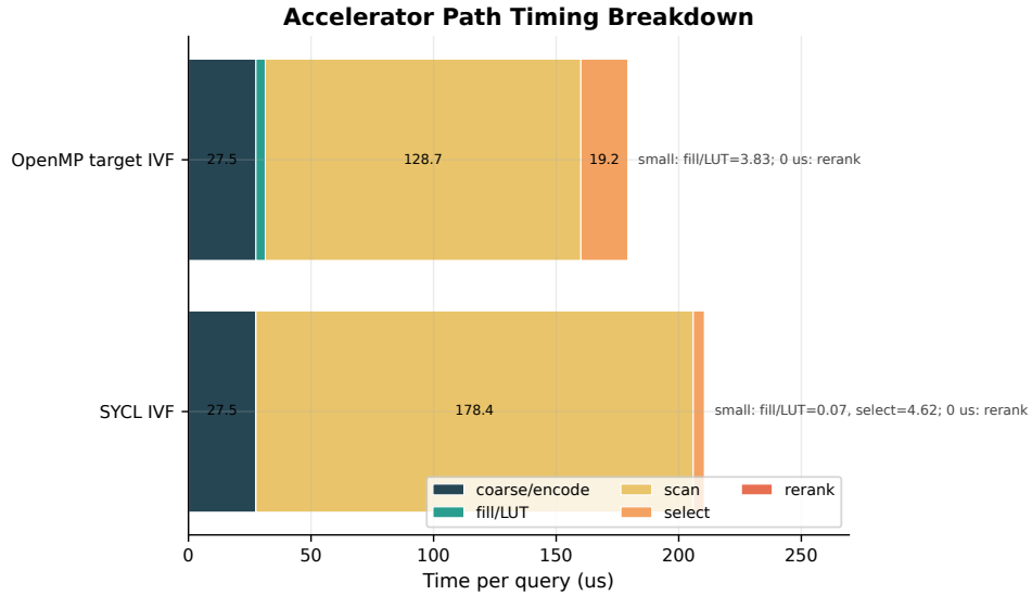
图 8: OpenMP target 与 oneAPI/SYCL 的阶段耗时分解。GPU 路径的主要开销集中在候选扫描和选择。
