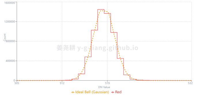
图 2. ILCE-7M3 红通道平场分布及高斯拟合 (6.46 码值)
