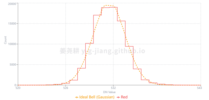
图 3. ILCE-7M3 红通道平场分布及高斯拟合 (17.12 码值)
