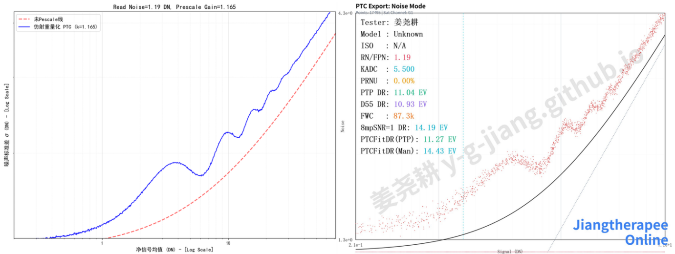
图 16. Prescaling 对 PTC 的模拟与实测对比
