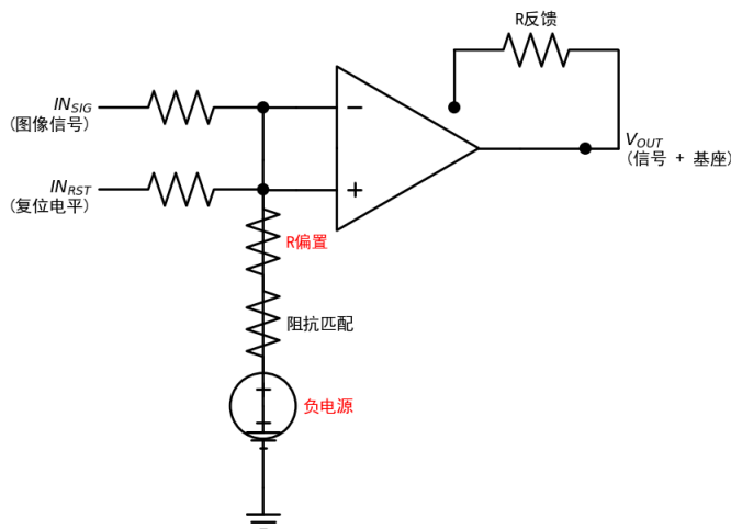
图 1. 黑电平基座与钳位机制示意
