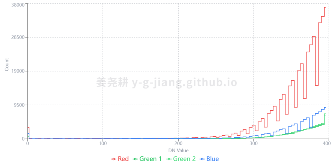
图 13. D850 黑位附近的断码分布
