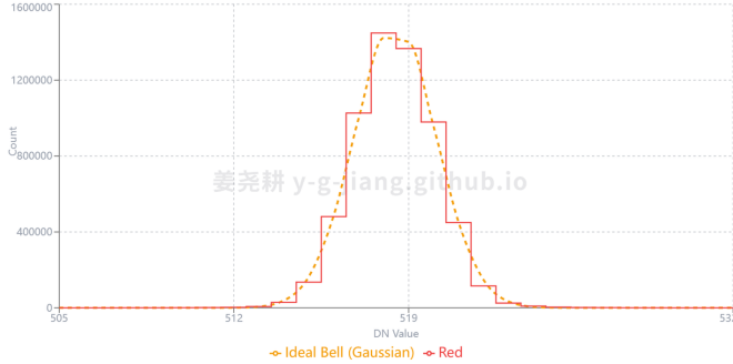
图 4. 平场能量谱 (堆叠平均)
