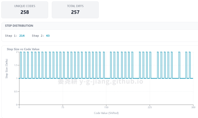
图 14. D850 高 ISO 下的码值粘连现象
