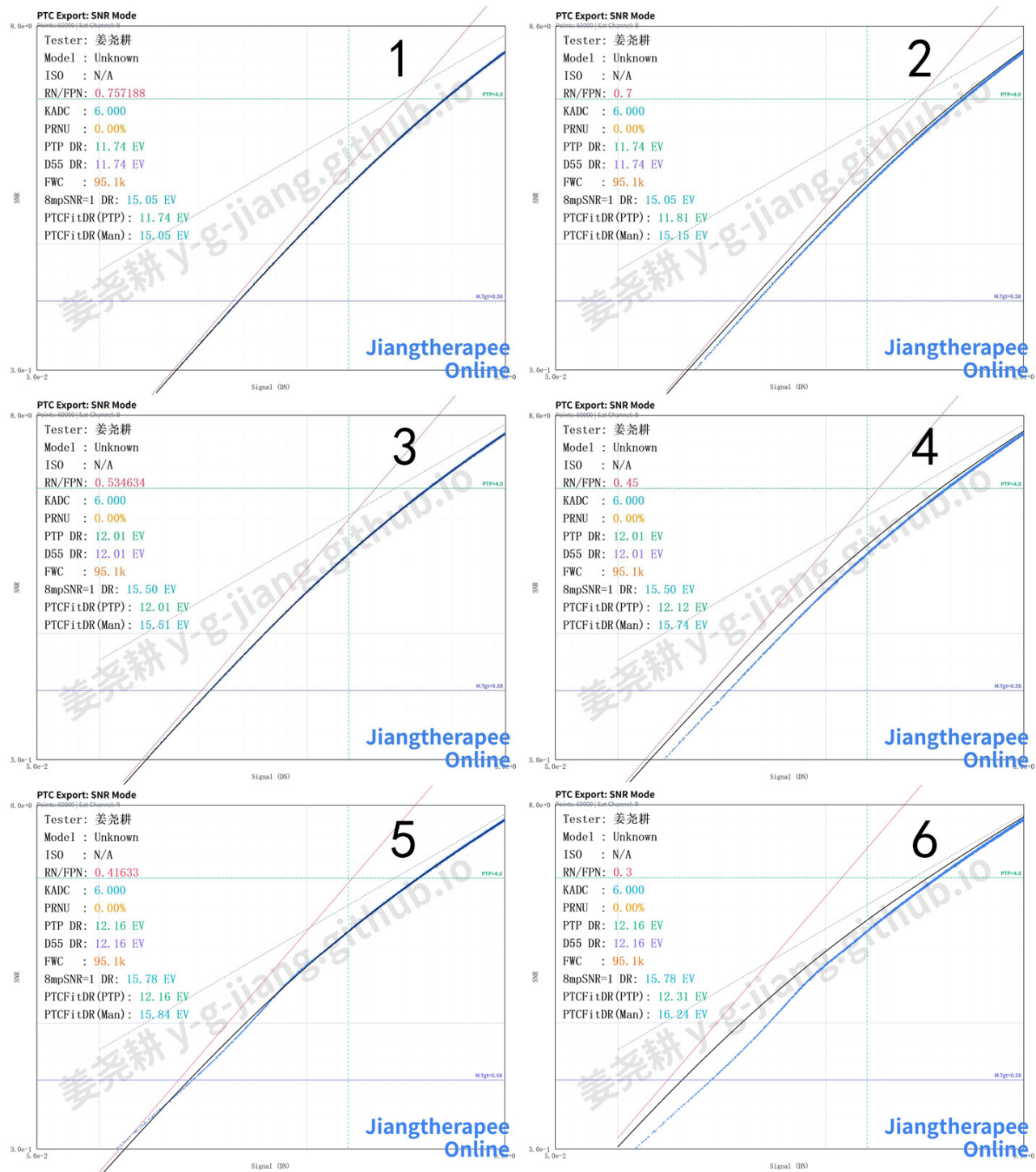
图 8. 三组读出噪声条件下的 PTC 拟合对比
