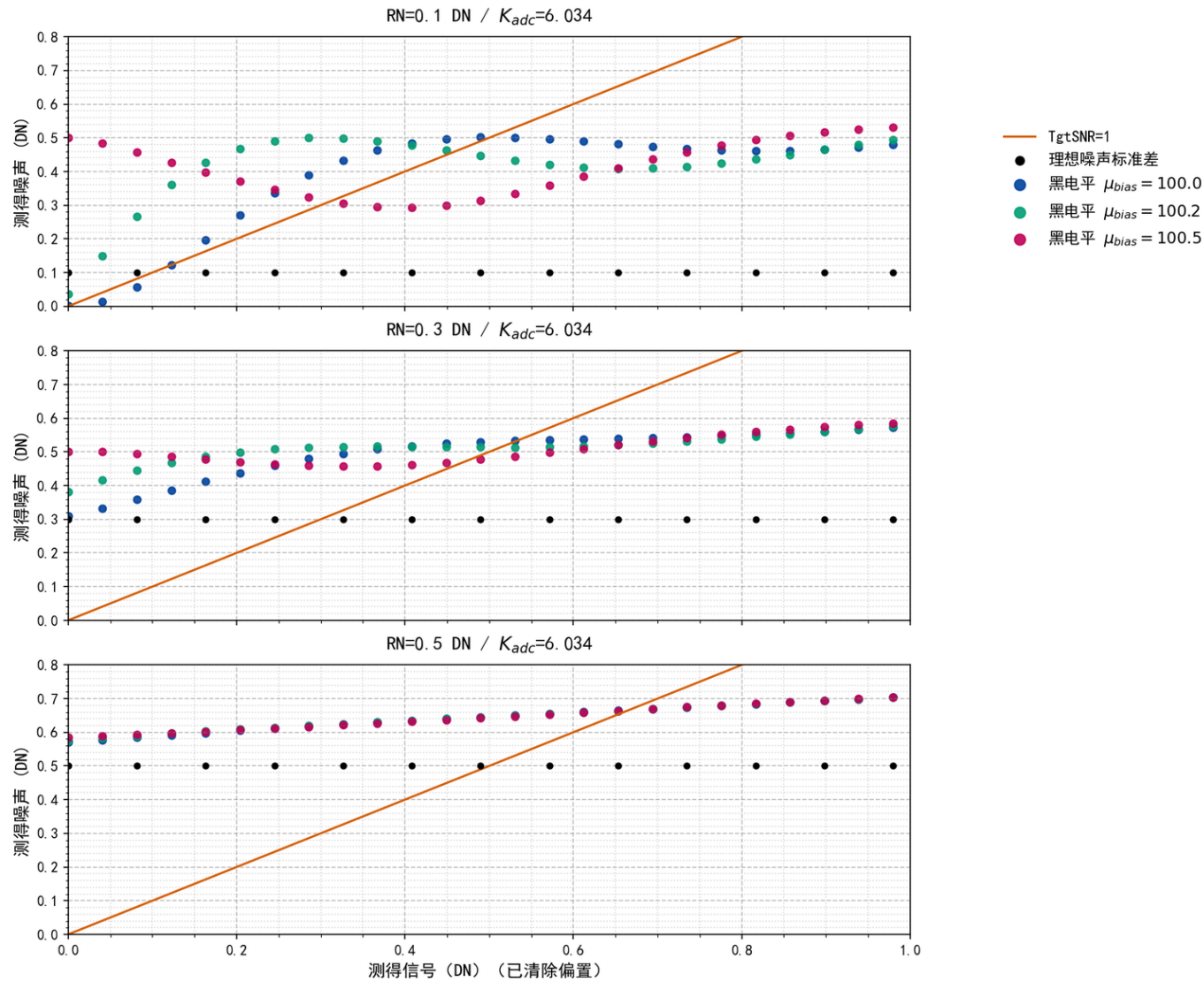
图 7. 偏移量化网格下的输出标准差曲线（均值组二）
