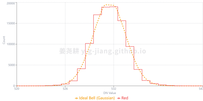
图 3. ILCE-7M3 红通道平场分布及高斯拟合 (17.12 码值)
