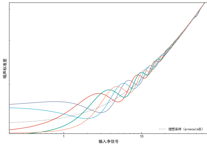
图 22. 不同乘减黑电平下的 DR 变化
