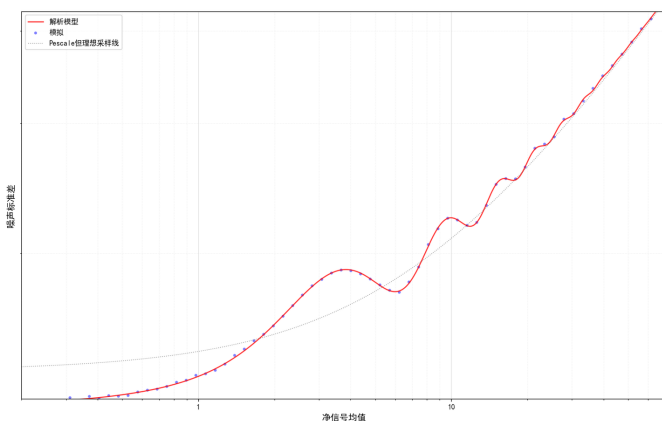
图 17. 非整数倍 prescaling 下的理论 PTC 震荡
