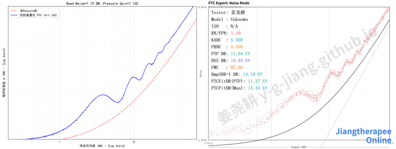
图 17. Prescaling 对 PTC 的模拟与实测对比
