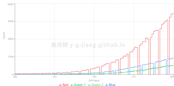
图 14. D850 黑位附近的断码分布
