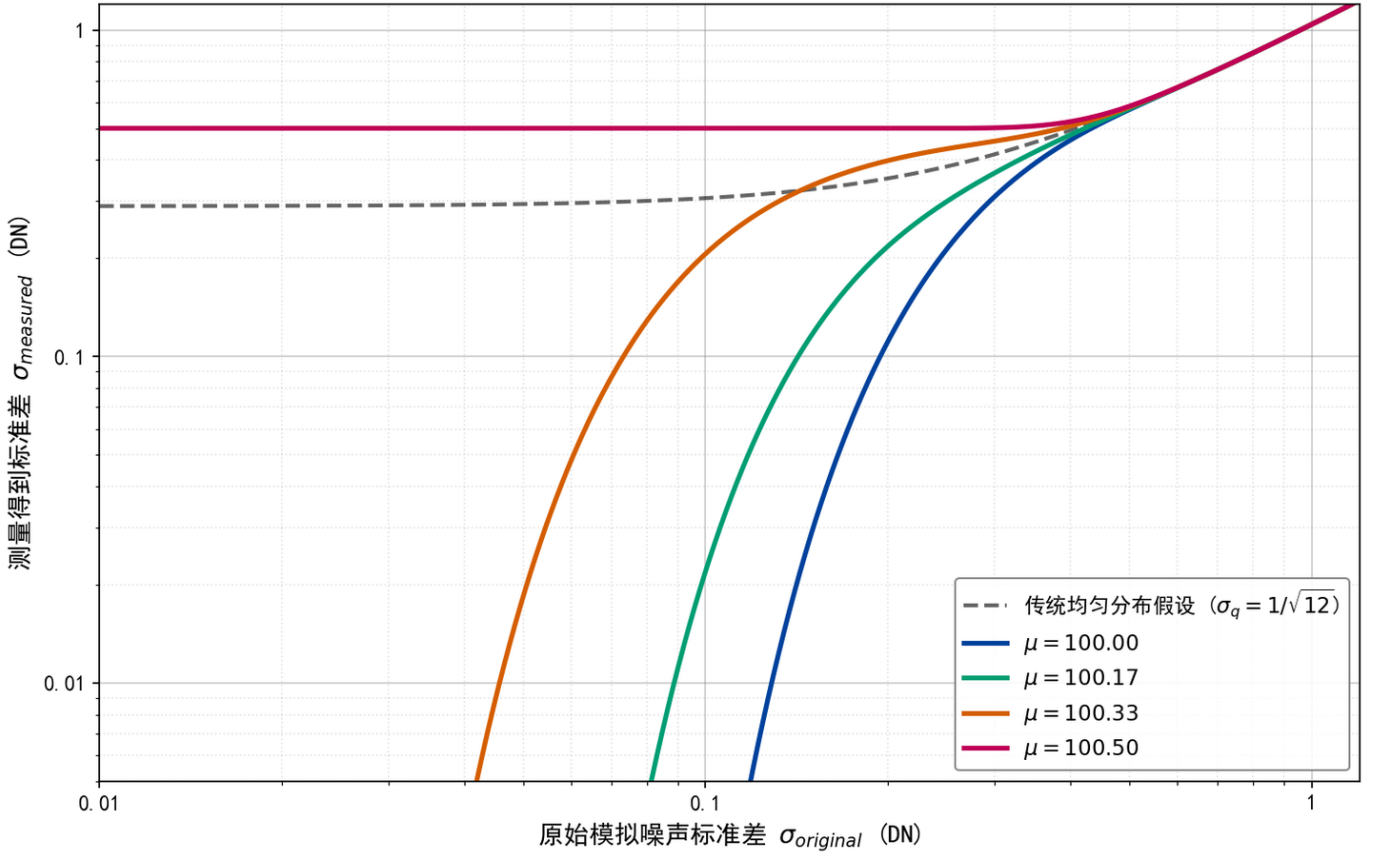
图 7. 偏移量化网格下的输出标准差曲线（均值组一）
