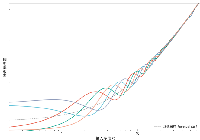
图 23. 不同乘减黑电平下的 DR 变化
