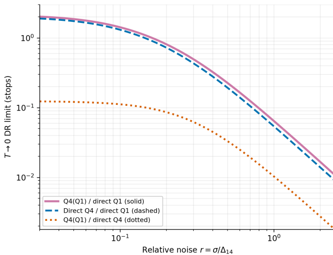
图 6. 两级 Q4(Q1) ties-to-even 的相位平均 MSE 与目标 SNR 参数 $T \rightarrow 0$ 时的 DR 极限。实线为两级链路相对直接 Q1 的总代价，虚线为直接 Q4 相对直接 Q1，点线为两级链路相对直接 Q4 的 tie 附加量；横、纵轴均为对数尺度。
