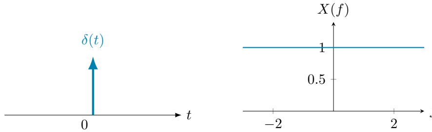
FIGURE 6 – TF de l'impulsion de Dirac \delta(t) (Propriété 3.3) : un spectre constant, X(f) = 1 pour tout f , donc toutes les fréquences présentes avec le même poids.
