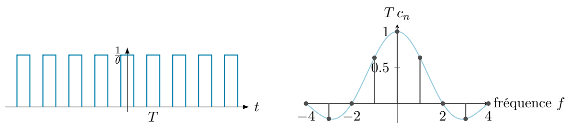
FIGURE 1 – Période T petite ( T = 1 , largeur d’impulsion \theta = 0.5 ). À gauche, le signal périodique dans le temps. À droite, les coefficients renormalisés Tc_n (bâtons noirs) de sa série de Fourier, peu nombreux et espacés de f_0 = 1/T , échantillonnent grossièrement la courbe enveloppe \theta \operatorname{sinc}(\pi f \theta) (en clair).
