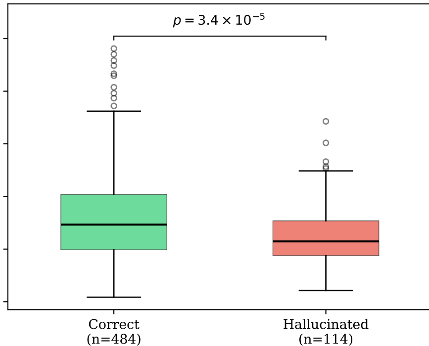
Llama 4 Maverick
