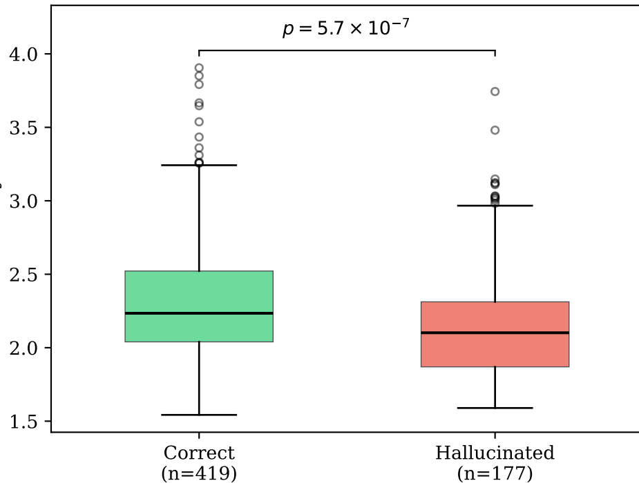
Mixtral 8x7B
