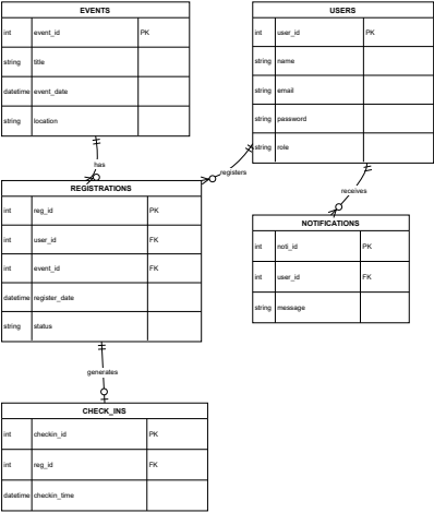
ERD (Mermaid)
