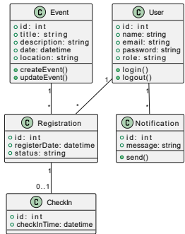
ERD (Mermaid)
